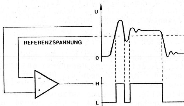
Abb. 1-2: Das zu speichernde Impulsmuster wird normiert und dann aus einer einstellbaren Logikschwelle gewonnen.
