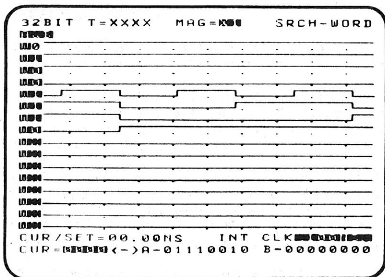
Abb. 4-28: Suchwort im Zeitdiagramm
