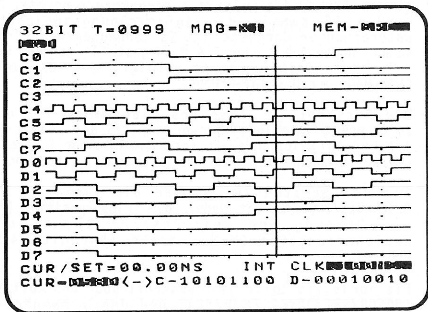
Abb. 4-19: Zeitdiagramm
