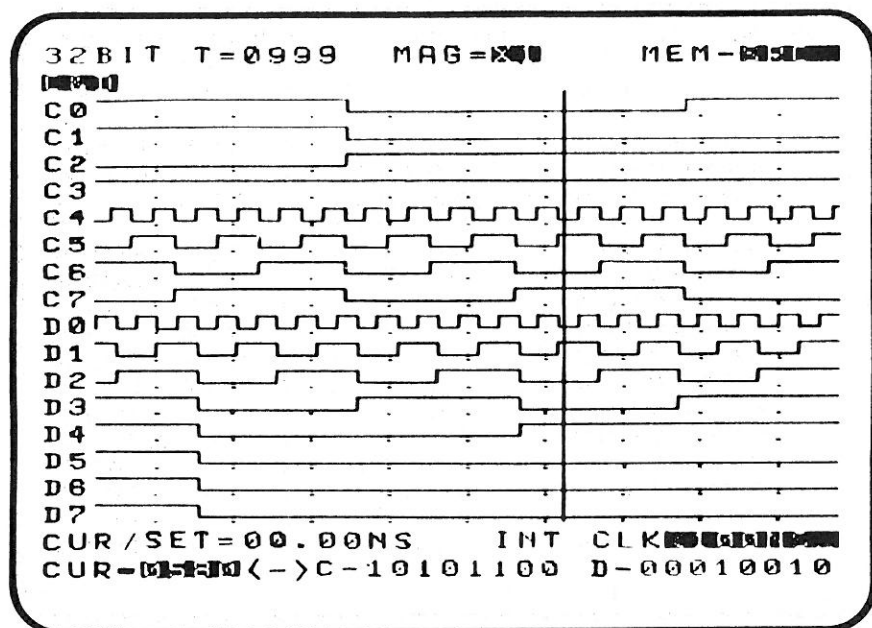
Abb. 6-13: Zeitdiagramm
