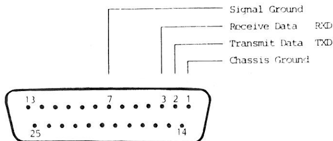
Abb. 5-1: RS-232-C-Anschlußbelegung
