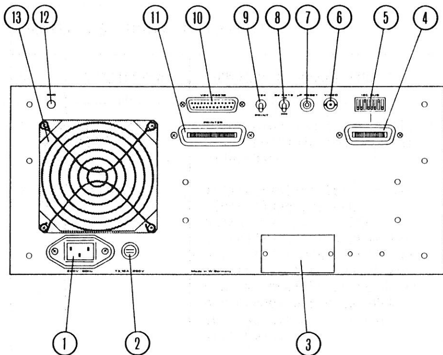
Abb. 3-10: Rückwand
