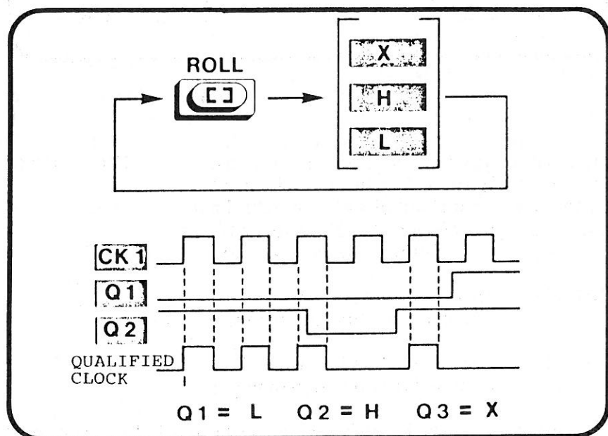
Abb. 4-7: Takt und Qualifizierer
