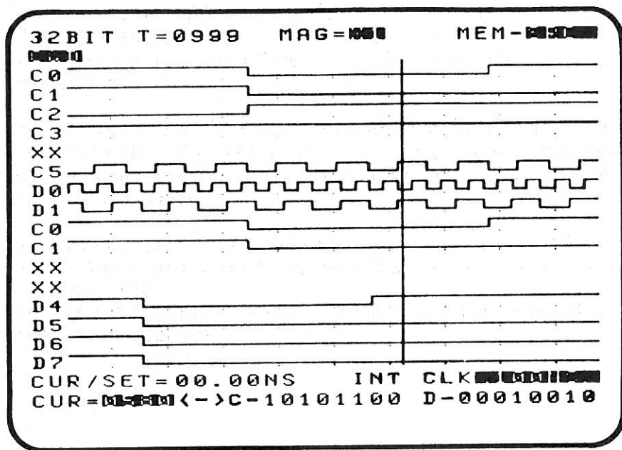
Abb. 4-20: Kanalanordnung im Zeitdiagramm
