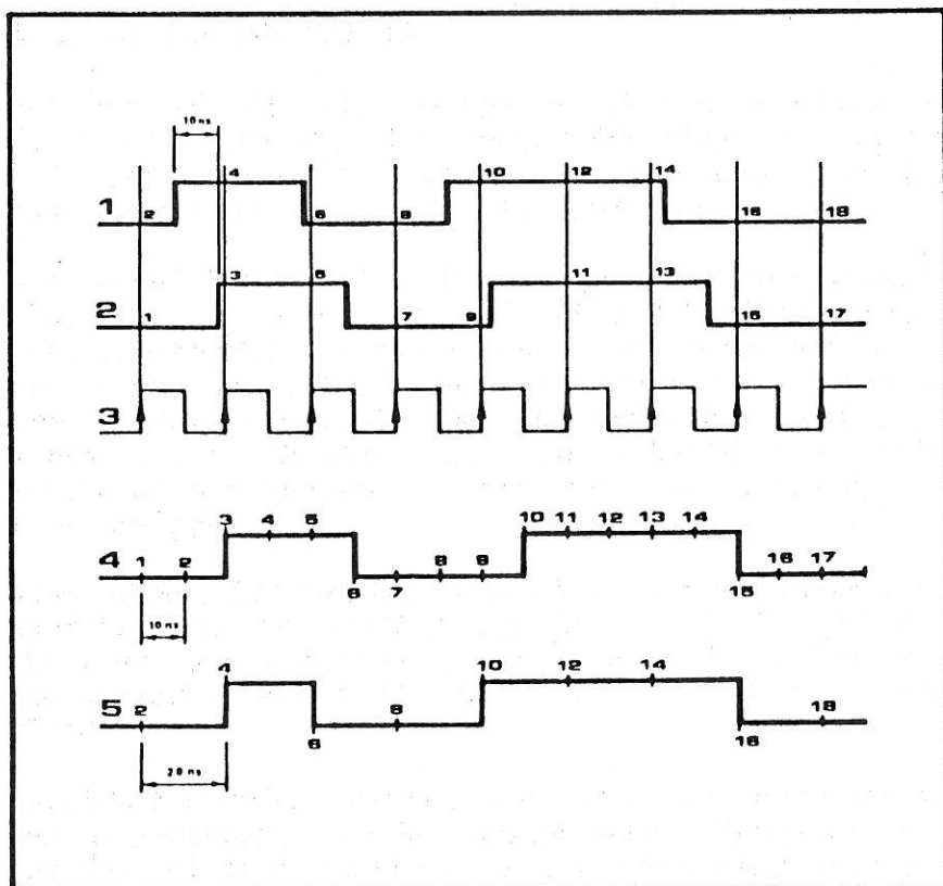
Abb. 4-33: Zum Funktionsprinzip der 100 MHz-Option
