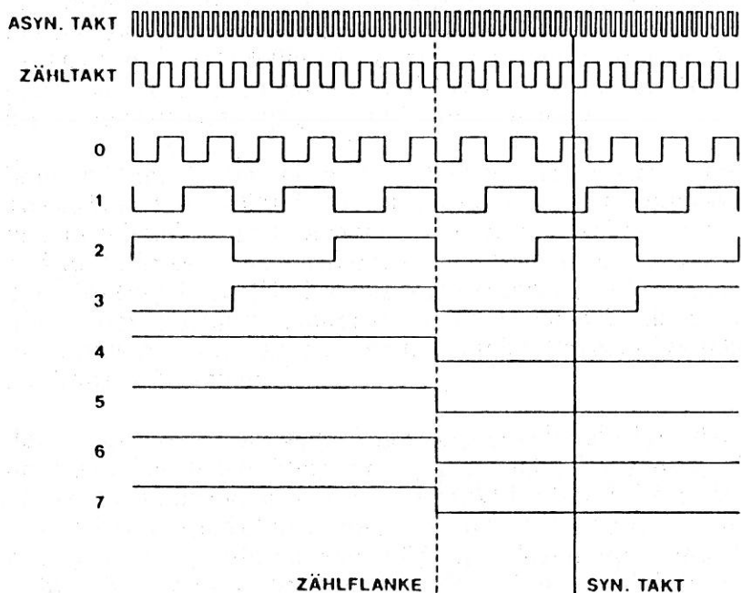
Abb. 1-4: Idealisiertes Zeitverhalten eines Binärzählers. Der Aufzeichnungstakt zur asynchronen und zur synchronen Abtastung ist jeweils mit angegeben
