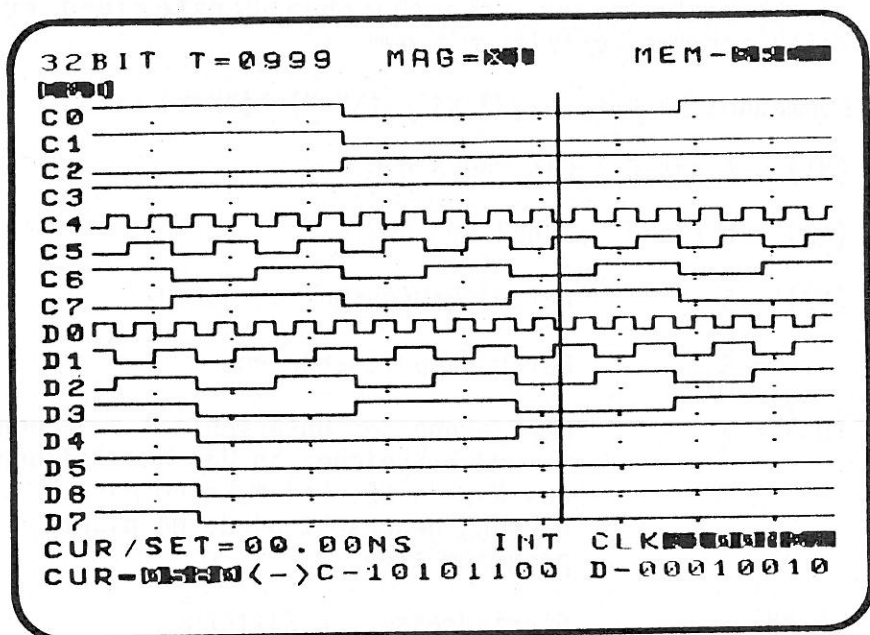
Abb. 5-13: Zeitdiagramm
