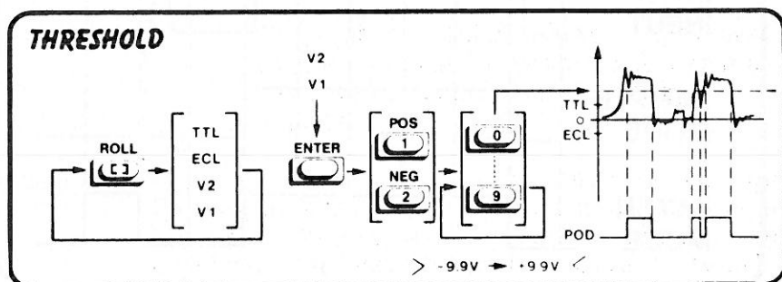
Abb. 4-5: Schwellwert
