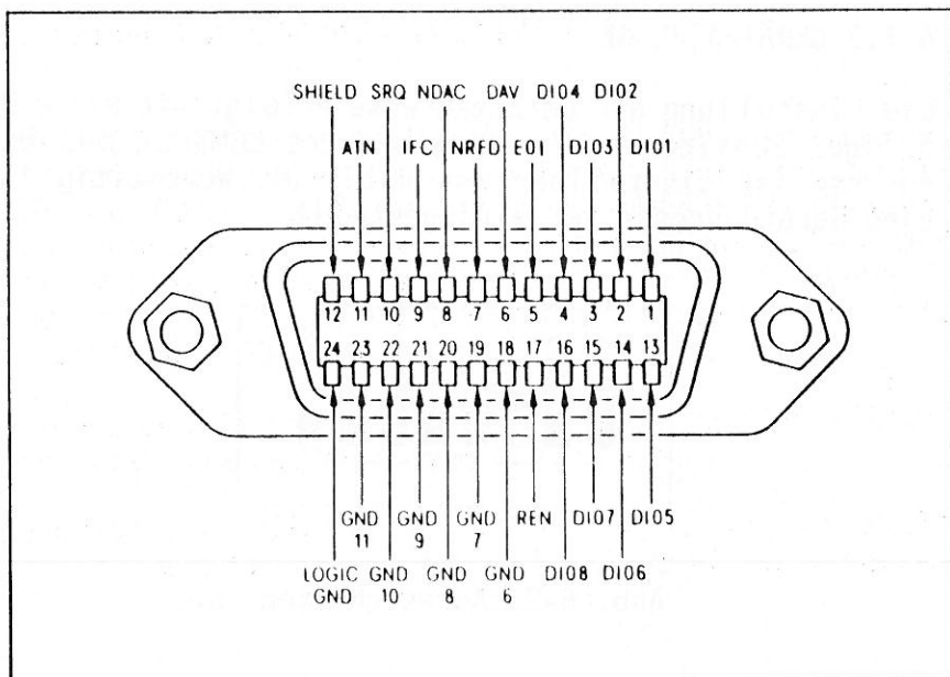
Abb. 6-1: GPIB Anschlußbelegung
