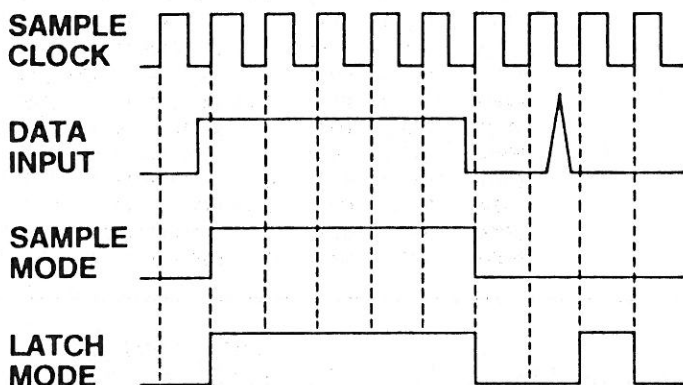
Abb. 1-7: Störimpulse zwischen zwei Abtastflanken werden in der normalen "Sample"-Betriebsart nicht erfasst. Die "Latch"-Betriebsart speichert den Störimpuls in einem separaten Glitch-Latch und zeigt ihn in der nächsten Taktperiode.
