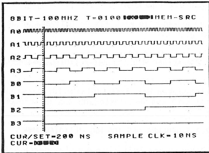
Abb. 4-34: 100 MHz-Zeitdiagramm
