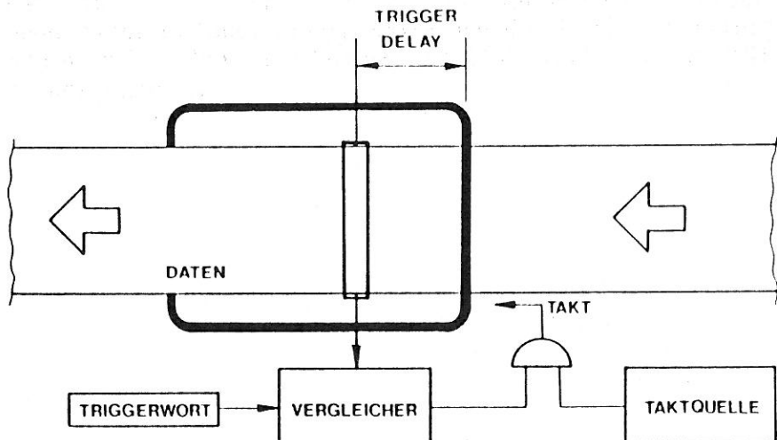
Abb. 4-14: Aufzeichnungsspeicher
