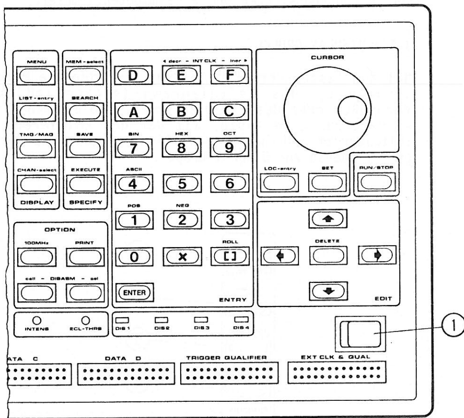
Abb. 3-1: Tastatur auf der Frontplatte
