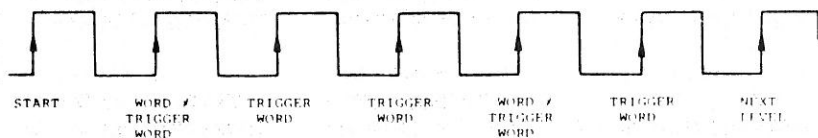
Fig. 4-10: Beispiel zur START-Funktion
