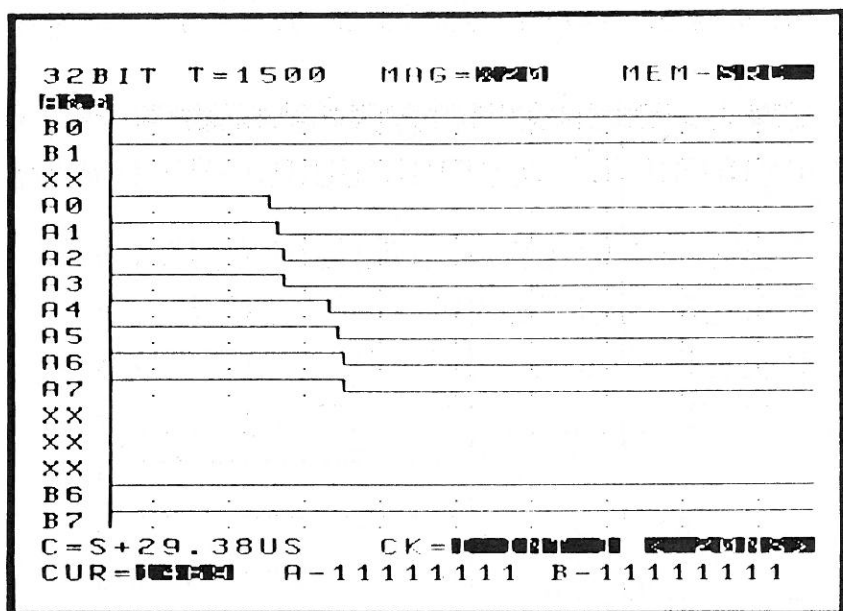
Abb. 1-5: Zeitdiagramm.
