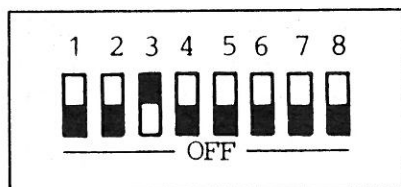
Abb. 6-2: Adressschalter
