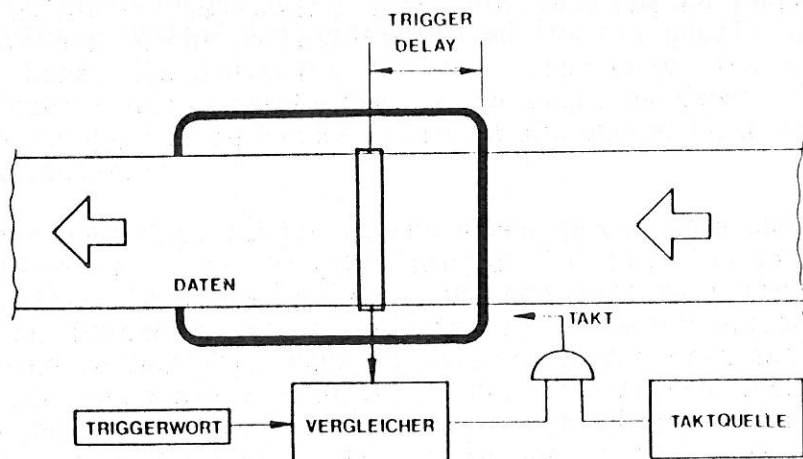
Abb. 1-1: Grundprinzip des Logikanalysators. Die Daten werden nach dem Prinzip eines Schieberegisters durch den Aufzeichnungsspeicher geschoben, bis die Triggerung die Aufzeichnung beendet.
