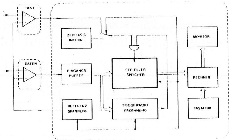
Abb. 1-3: Das stark vereinfachte Blockschaltbild eines Logikanalysators
