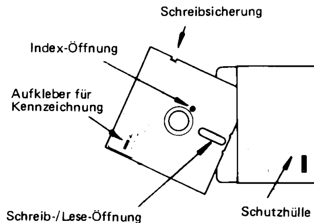
Abb. 3.1 Diskette
