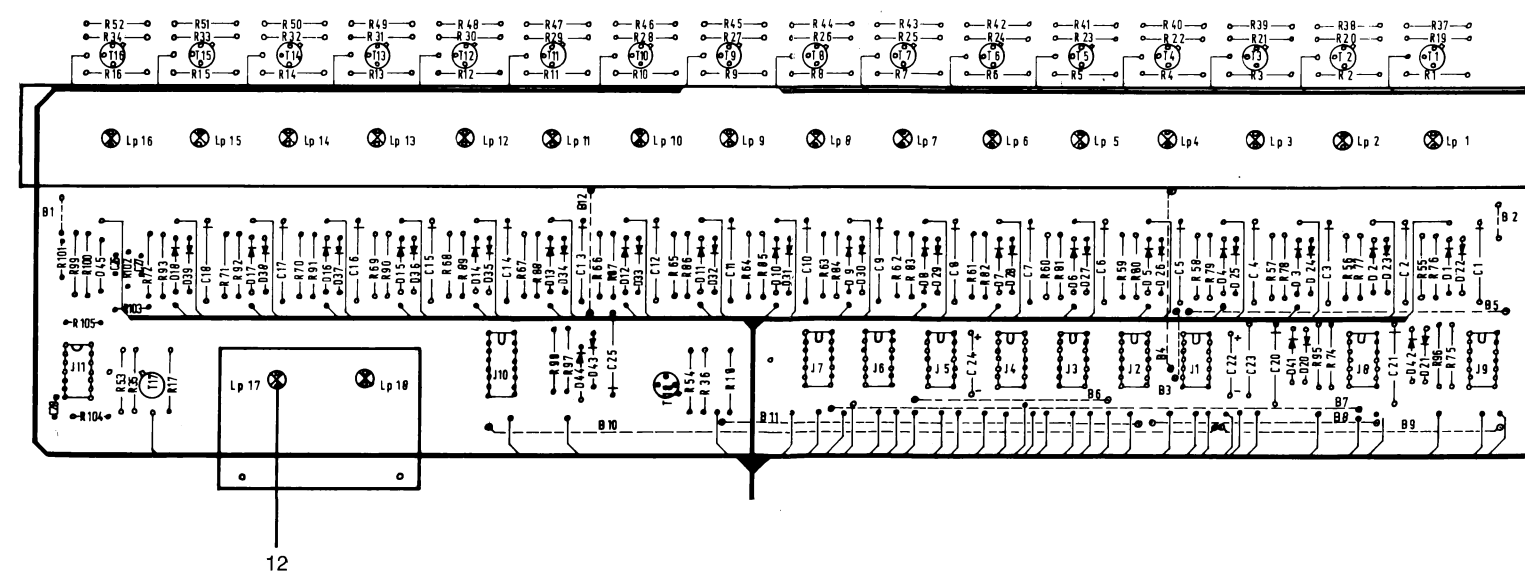
Bedienfeld, Schrank Abb. 2
