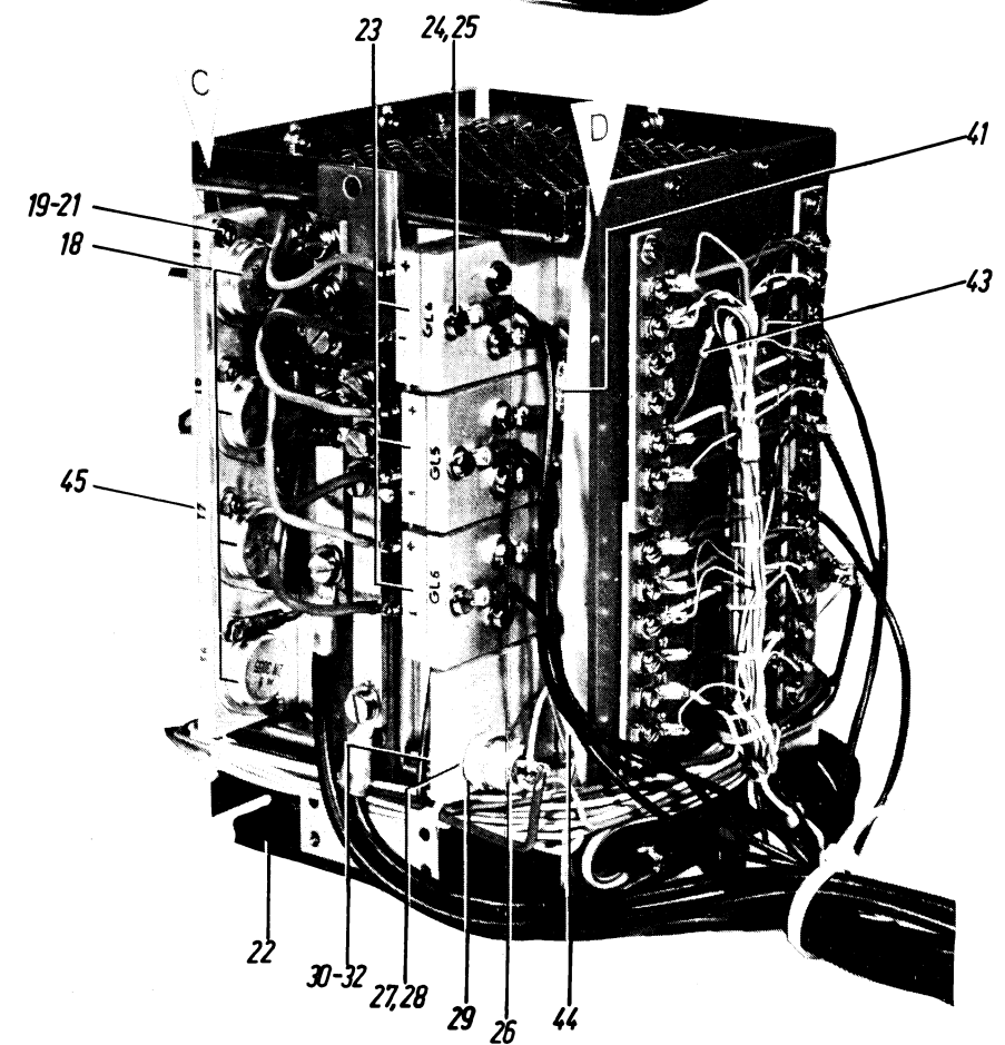
Kühlsäule + 12/-12V Abb. 1.2
