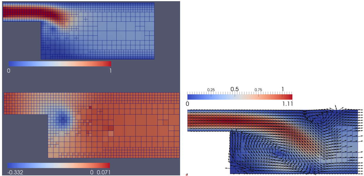
(a) Zeitpunkt t = 0,54 , oben: Geschwindigkeitsfeld, Farbgebung nach Betrag der Geschwindigkeit, unten: Druckfeld
