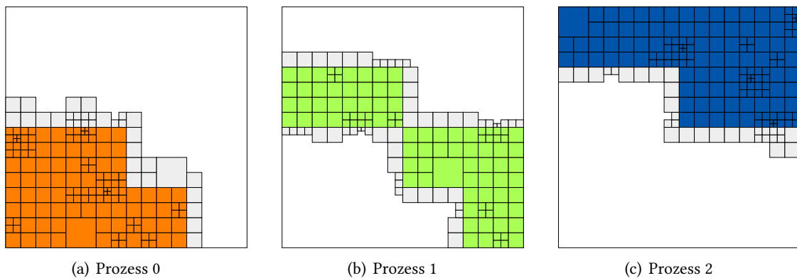
Abbildung 2.11. Kompletter balancierter Quadtree, aufgeteilt auf 3 Prozesse mit Ghost-Quadranten in grau.
