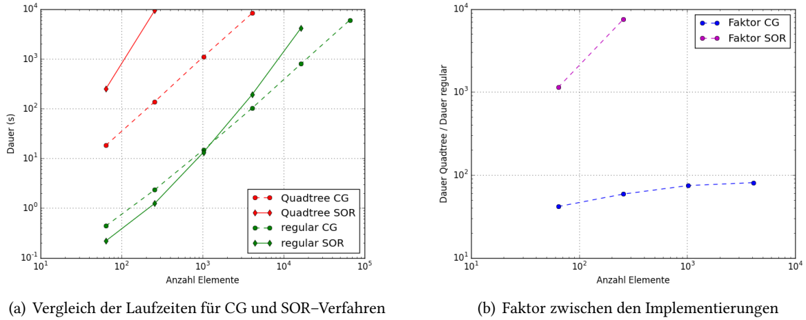
Abbildung 4.11. Vergleich der Laufzeit bei serieller Ausführung zwischen der Implementierung mit Quadtrees und der direkten Implementierung als reguläres Gitter
