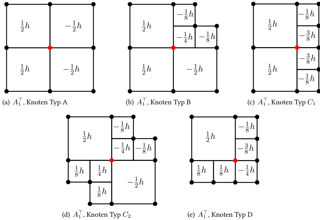
Abbildung A.5. Differenzensterne für den Operator A_1^\top für die verschiedenen Knotentypen
