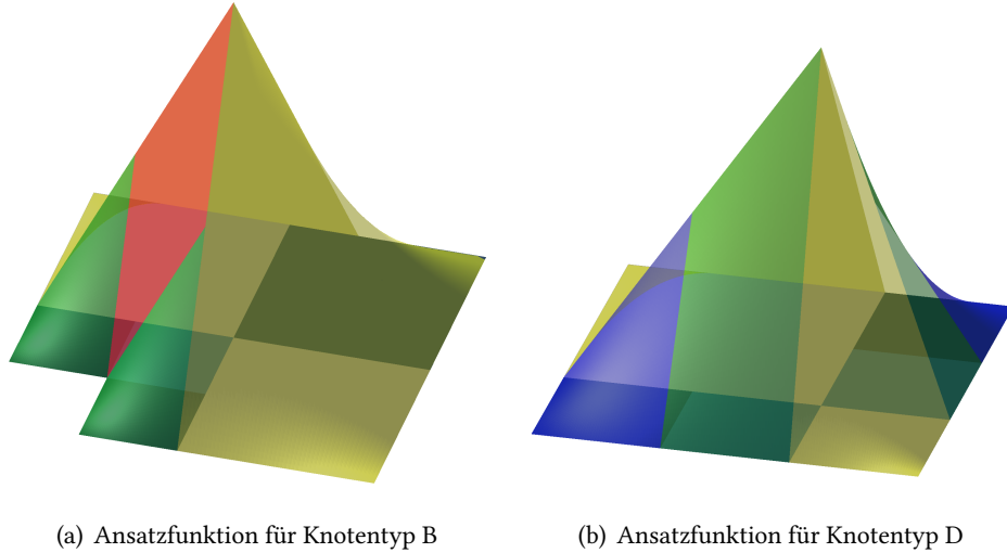
Abbildung 2.19. Ansatzfunktionen \phi_A(\mathbf{x})
