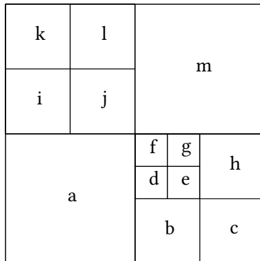
(a) Quadtree als Zerlegung eines Gebiets
