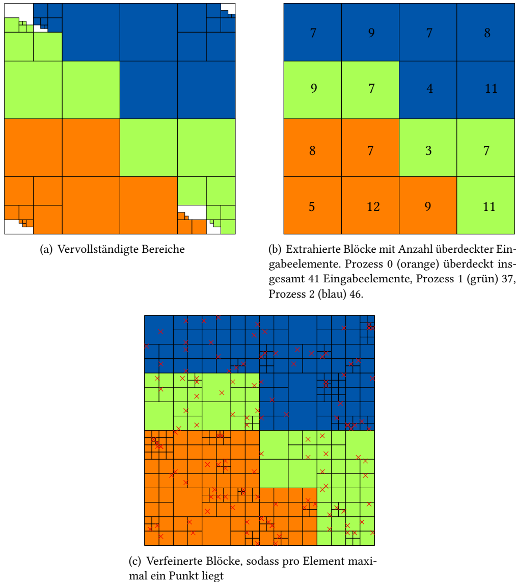
Abbildung 2.6. Erzeugung von Blöcken und anschließende Verfeinerung
