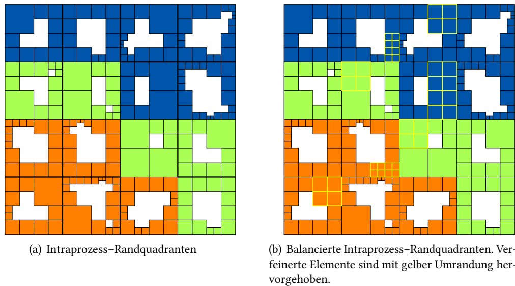
Abbildung 2.8. Intraprozess–Grenzquadranten. Die Grenzen zwischen Blöcken auf einem Prozess sind mit dickerer Linie hervorgehoben.
