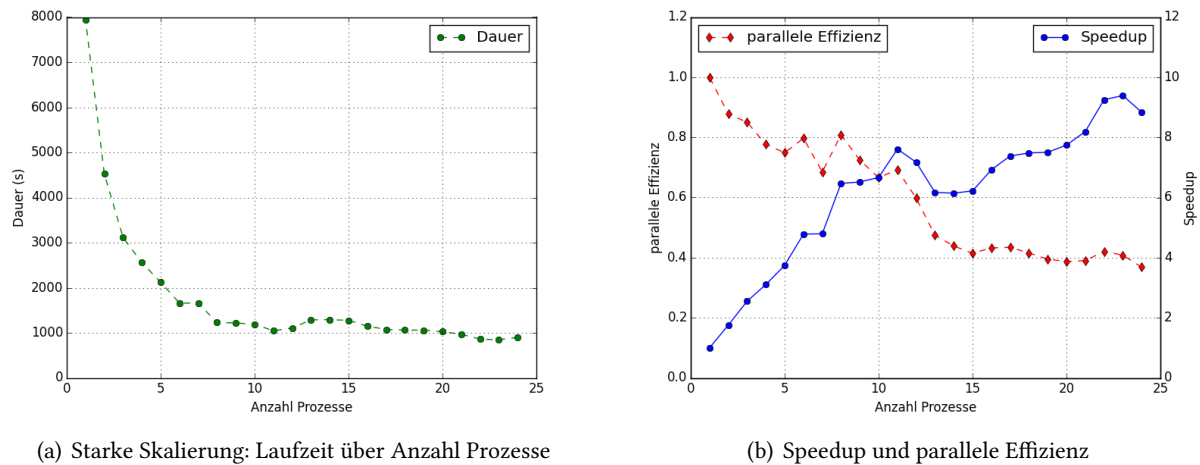
Abbildung 4.6. Untersuchung der starken Skalierung
