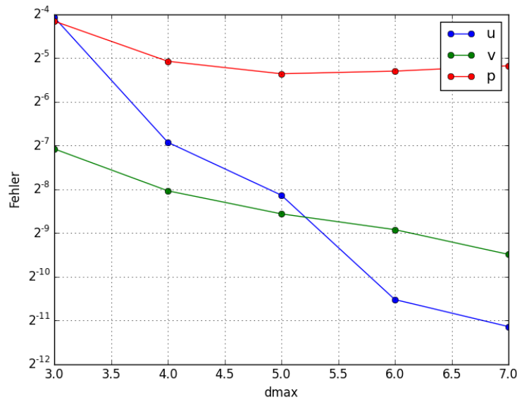
Abbildung 4.13. Konvergenzanalyse der Poiseuilleströmung für verschiedene Gitterweiten
