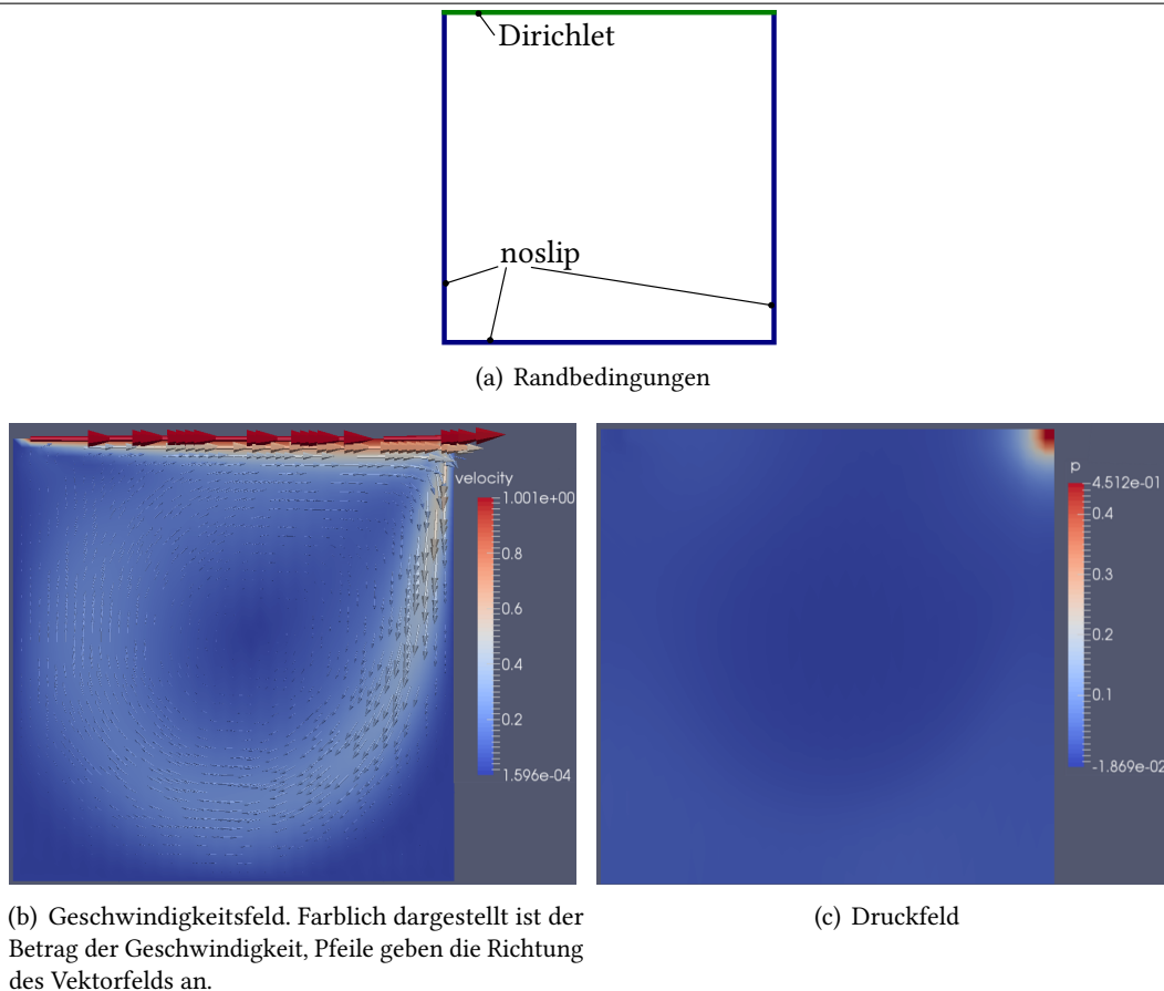
Abbildung 3.2. Szenario „driven cavity“
