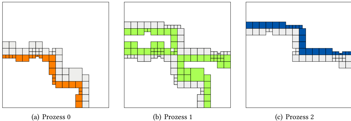
Abbildung 2.10. Balancierte Interprozess-Grenzquadranten. In Farbe sind die jeweiligen Elemente dargestellt, die der Prozess besitzt, in grau die von anderen Prozessen erhaltene Grenzquadranten, die zur Balancierung notwendig sind.
