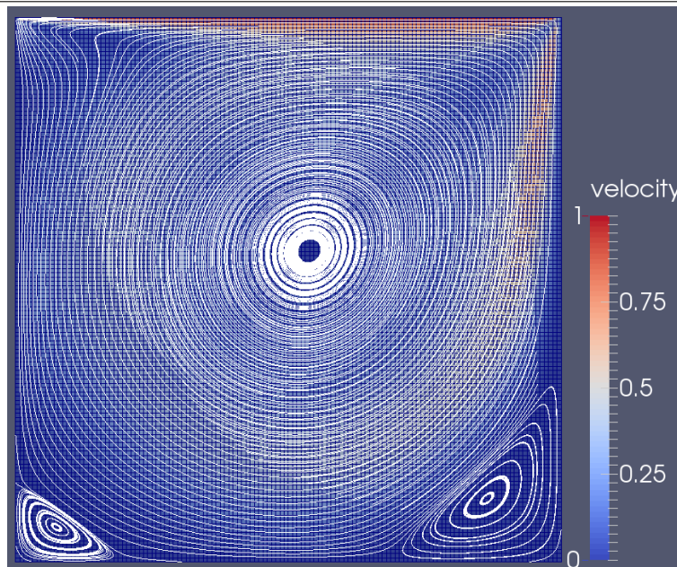
Abbildung 4.5. Geschwindigkeit und streamlines für „driven cavity“, t = 20 , Re = 1000 , L_1 = L_2 = 1 , d_{\max} = 7
