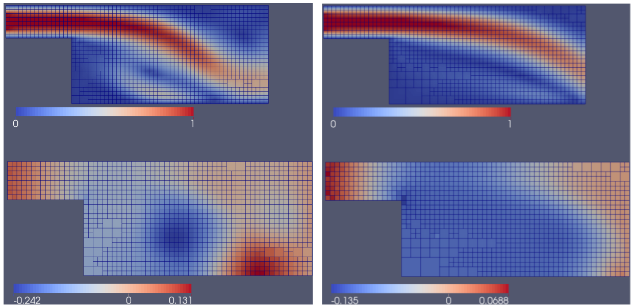
(c) Zeitpunkt t = 2,77 , Oben: Geschwindigkeitsfeld, Farbgebung nach Betrag der Geschwindigkeit, unten: Druckfeld
