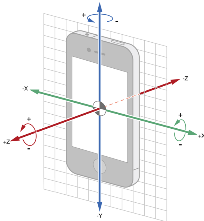
Abbildung 2.1.: Die Abbildung zeigt die Messachsen und -richtungen eines Beschleunigungssensors und die Rotationsrichtung eines Gyroskops in einem Smartphone. Smartphone. 9
