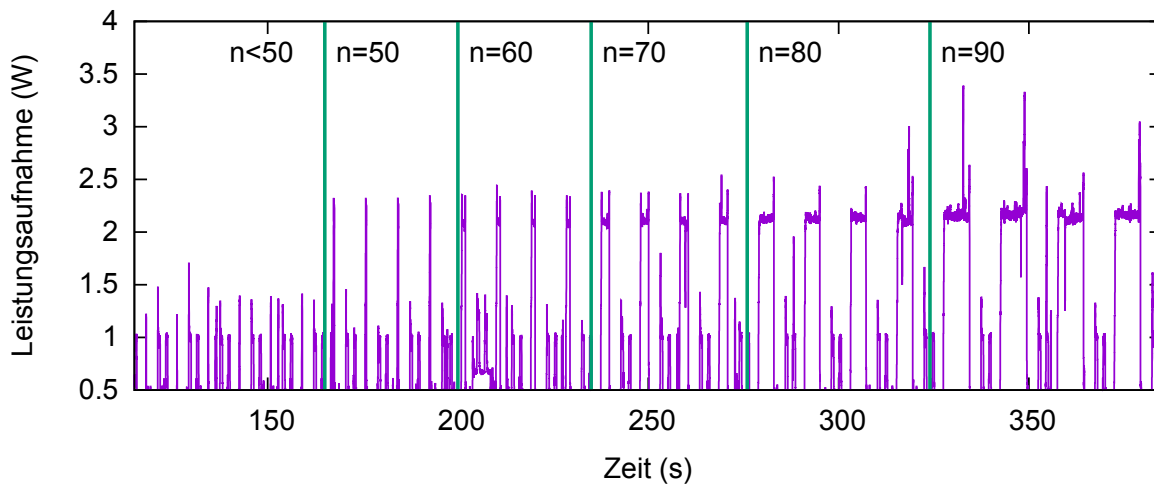
Abbildung 7.4: Leistungsaufnahme im zeitlichen Verlauf des Profilings; die vertikalen Linien grenzen Ausführungen verschiedener Qualitätsparameter voneinander ab
