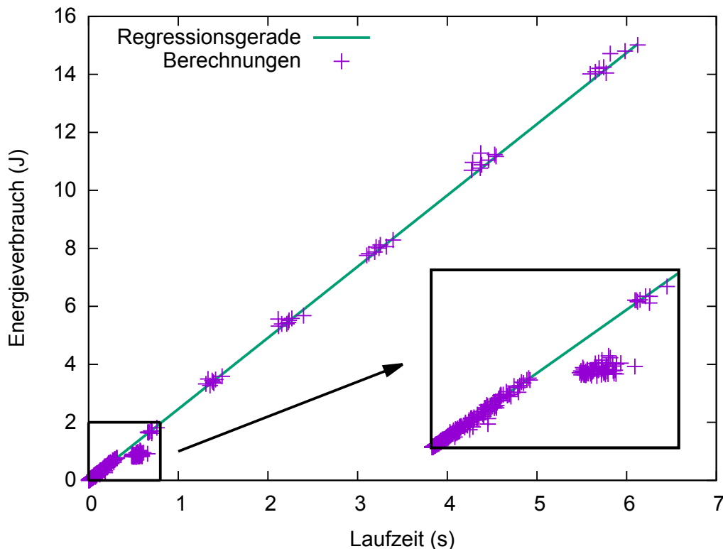
Abbildung 7.8: Abbildung der Laufzeiten verschiedener Ausführungen der Canny Edge Detection auf den dazugehörigen Energieverbrauch, mit Regression f(x) = mx
