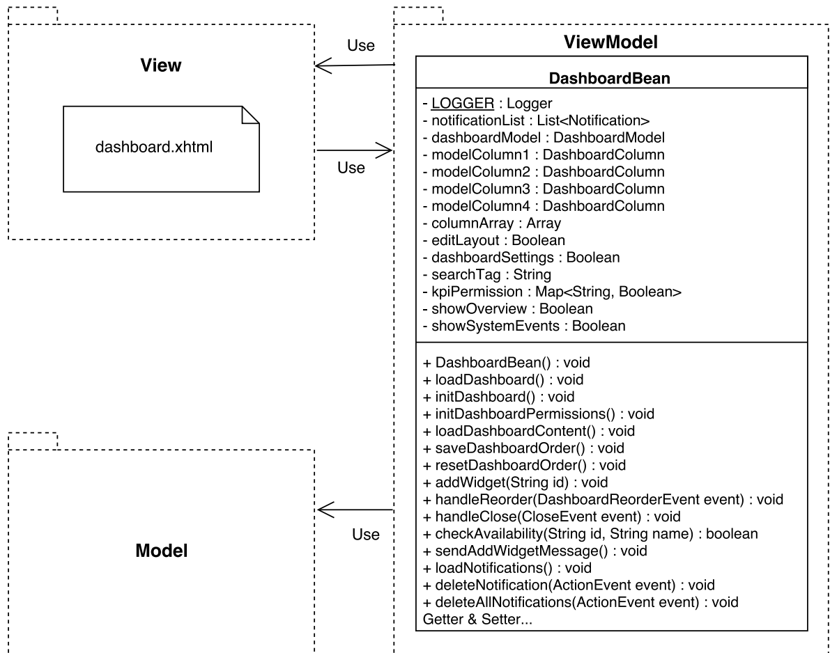
Abbildung 5.4: UML-Diagramm zu Dashboard-Facelet und DashboardBean
