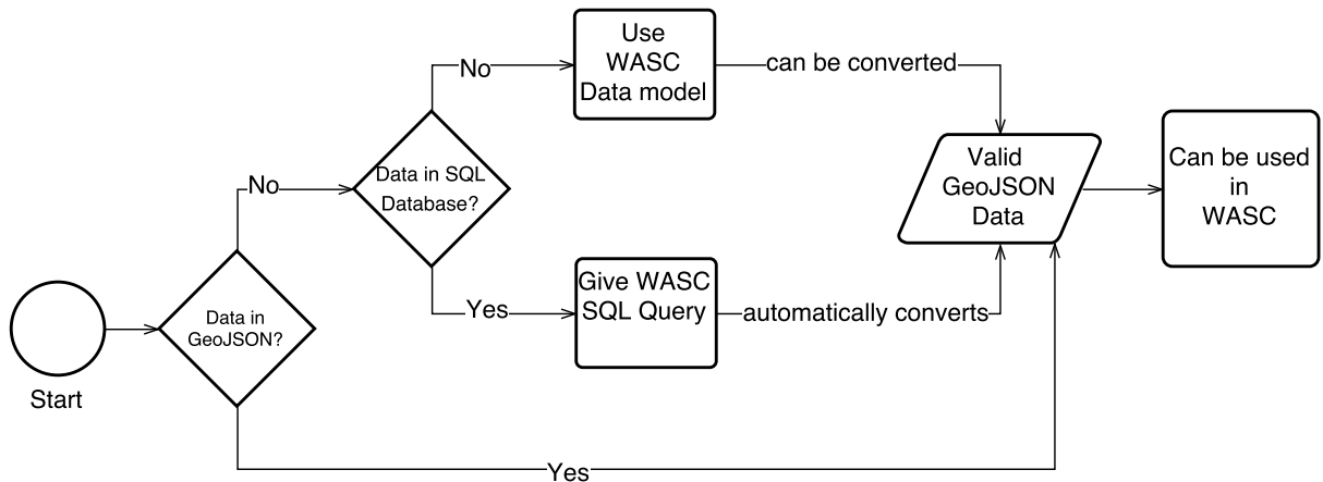
Abbildung 5.3.: Ablaufdiagramm für einen Datenimport in WASC. Eigene Abbildung.
