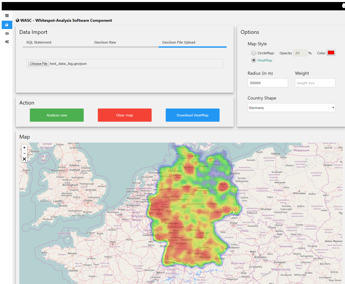
Abbildung 5.2.: Momentaufnahme von der WASC Frontendschnittstelle. Abgebildet ist der Inhalt des 'Analysis' Menüpunktes, in dem ein Testdatensatz hochgeladen wurde. Es wurde die Intensitätsübersicht als Ausgabe gewählt. Die anderen Menüpunkte sind als minimierte Symbole oben links im Bild zu sehen. Eigene Abbildung.
