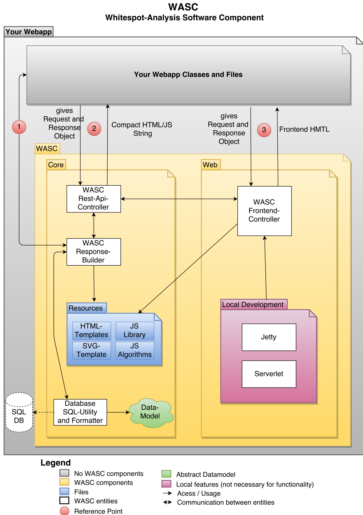
Abbildung 5.1.: Komponentendiagramm von WASC. Eigene Abbildung.
