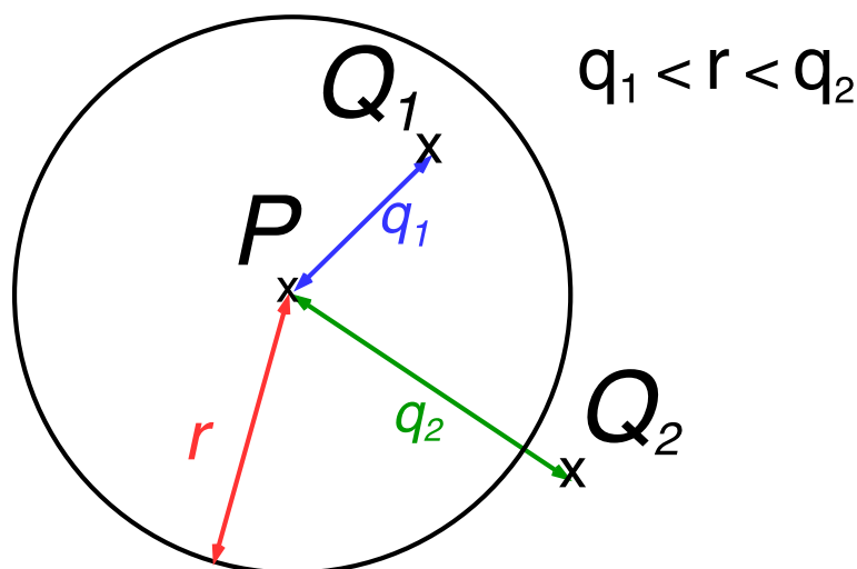
Abbildung 3.1.: Darstellung vom Umkreis um Punkt P mit zwei Punkte Q_1 und Q_2 . Die Längen der farbigen Geraden ( r , q_1 , q_2 ) sind wie folgt geordnet 'q1 kleiner r kleiner q2'. Eigene Abbildung.
