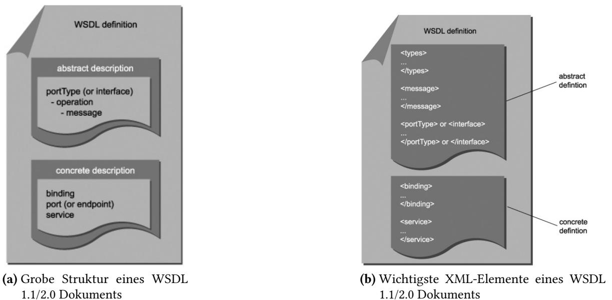
Abbildung 2.11: Struktur eines WSDL Dokuments [Erl05]
