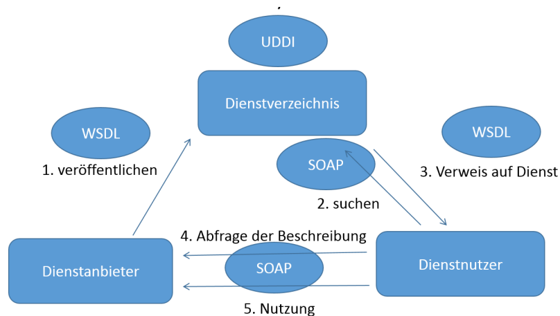
Abbildung 2.4: Das SOA-Dreieck in einer Realisierung mit Webservices [Dos05]
