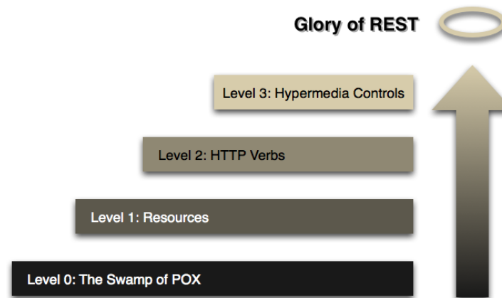
Abbildung 2.10: Level des Richardson Maturity Models [Fow10]
