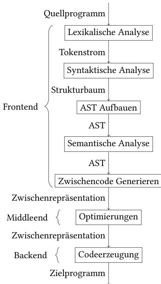
Abbildung 3.1.: Zu sehen ist, wie der Programmcode die unterschiedlichen Teile eines Compiler durchläuft und welche Repräsentation er annimmt.
