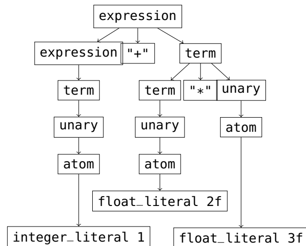
Abbildung 3.2.: (Links) Eine kleine Beispielgrammatik für arithmetische Ausdrücke. Die Symbole integer_literal und float_literal , sowie alles in Anführungszeichen sind Terminalsymbole. Die Grammatik stellt sicher, dass Operationen mit höherer Präzedenz im resultierenden Strukturbaum zusammen gehören. Operatorpräzedenz ist also schon Teil der Syntax und nicht erst der Semantik. Außerdem werden Klammern und das unäre Minus richtig gruppiert. Diese Grammatik besteht aus Regeln die mit Semikola beendet werden. Jede Regel beginnt mit dem Nichtterminalsymbol, welches durch die Regel definiert wird. Danach folgt ein Doppelpunkt und eine oder mehrere, durch vertikale Striche getrennte, Produktionen für dieses Nichtterminalsymbol. (Rechts) Der Strukturbaum des Ausdrucks 1 + 2f * 3f auf den die syntaktische Analyse mit der Grammatik links angewendet wurde. Die Terminalsymbole sind die drei Zahlen und die beiden Operatoren. Das nachstehende f an den Zahlen bedeutet, dass es sich um floats handelt. Das Startsymbol muss in diesem Fall expression sein. Wie hier zu sehen ist, ist der resultierende Strukturbaum unnötig groß, zusammenhängende Teile sind weit auseinander. Wie während der Bearbeitung dieser Arbeit festgestellt wurde, macht das die Verarbeitung schwer.
