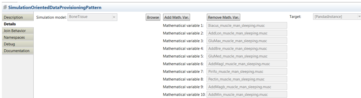
Abbildung 4.2: Property Section des simulationsorientierten Data Provisioning Patterns
