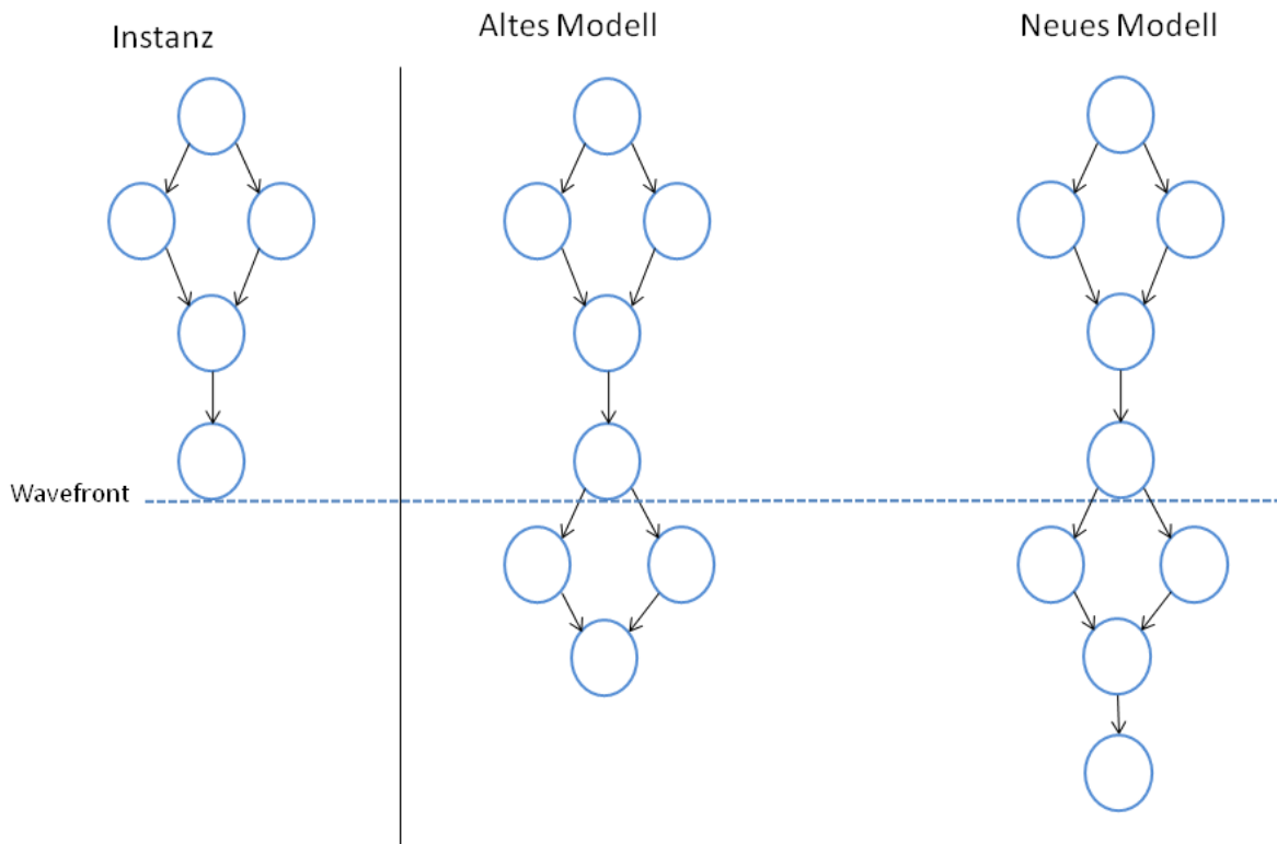
Abbildung 5.1: Wavefront einer Instanz Quelle: [Sch11]
