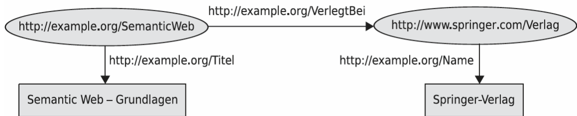
Abbildung 2.11: Einfacher RDF Graph mit Literalen. Quelle: [HKRS07]
