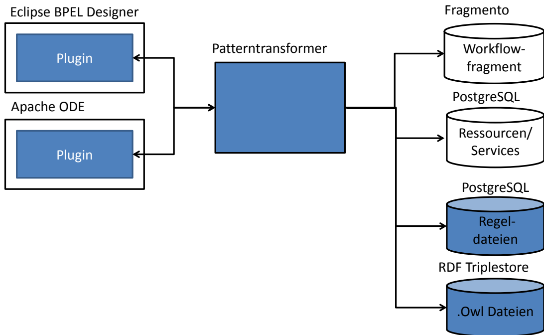
Abbildung 6.1: Entwurf der neuen Patterntransformation
