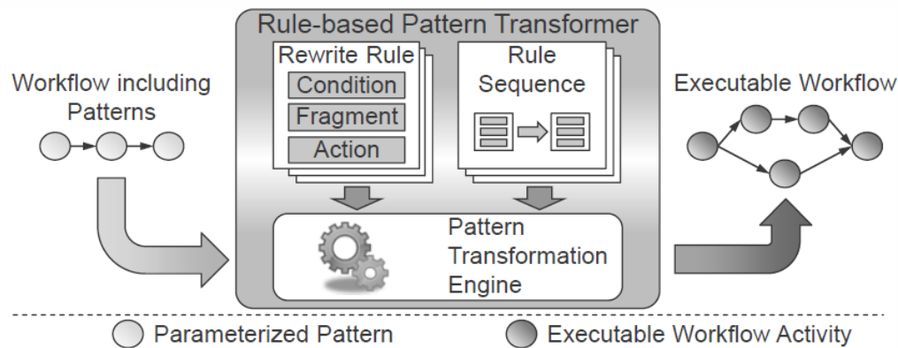
Abbildung 2.10: Modell der Transformation von Datenmanagementpatterns vgl. [RSM14b]
