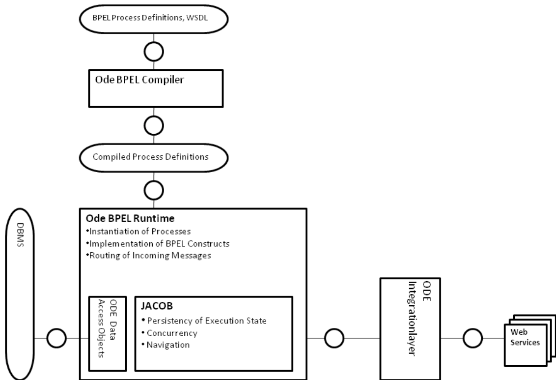
Abbildung 2.7: Apache ODE Architektur Quelle: [ode]
