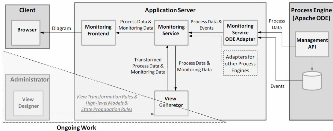
Abbildung 9.1: generische Architektur für das Monitoring von Geschäftsprozessen in mehreren Abstraktionsschichten Quelle: [SLL11a]
