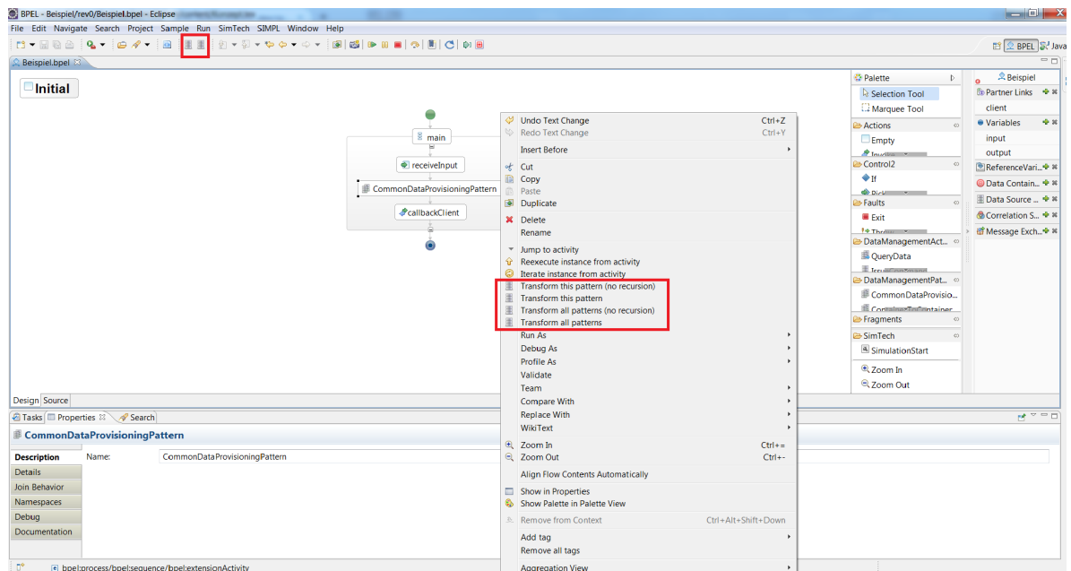
Abbildung 7.1: Optionen der Patterntransformation innerhalb der Eclipse BPEL Entwicklungsumgebung
