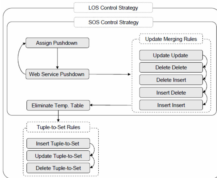
Abbildung 9.4: Kontrollstrategien der Optimierungssphären Quelle: [VSS + 07]
