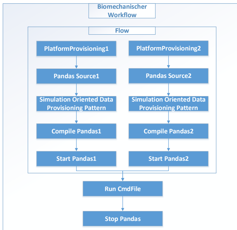
Abbildung 3.4: Aufbau des biomechanischen Workflows Quelle: [Boh14]
