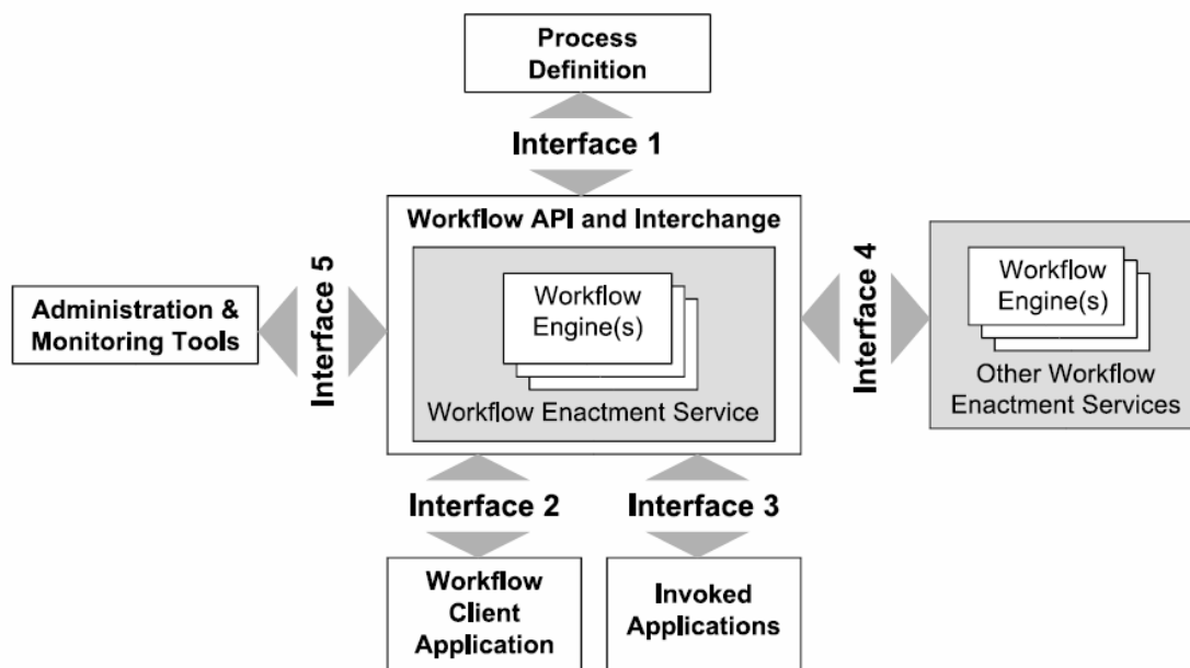
Abbildung 2.6: Referenzmodell eines WfMS Quelle: [LR00]
