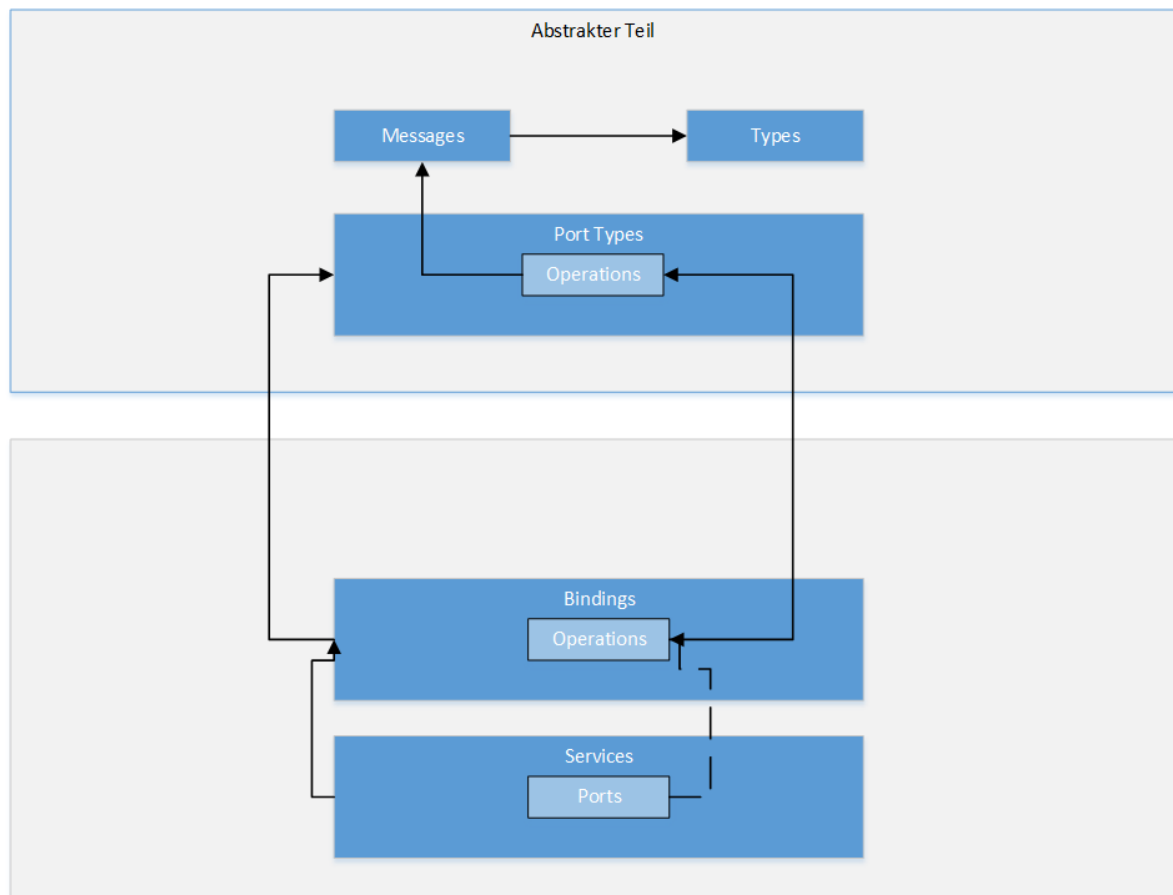
Abbildung 2.3: Aufbau einer WSDL Datei
