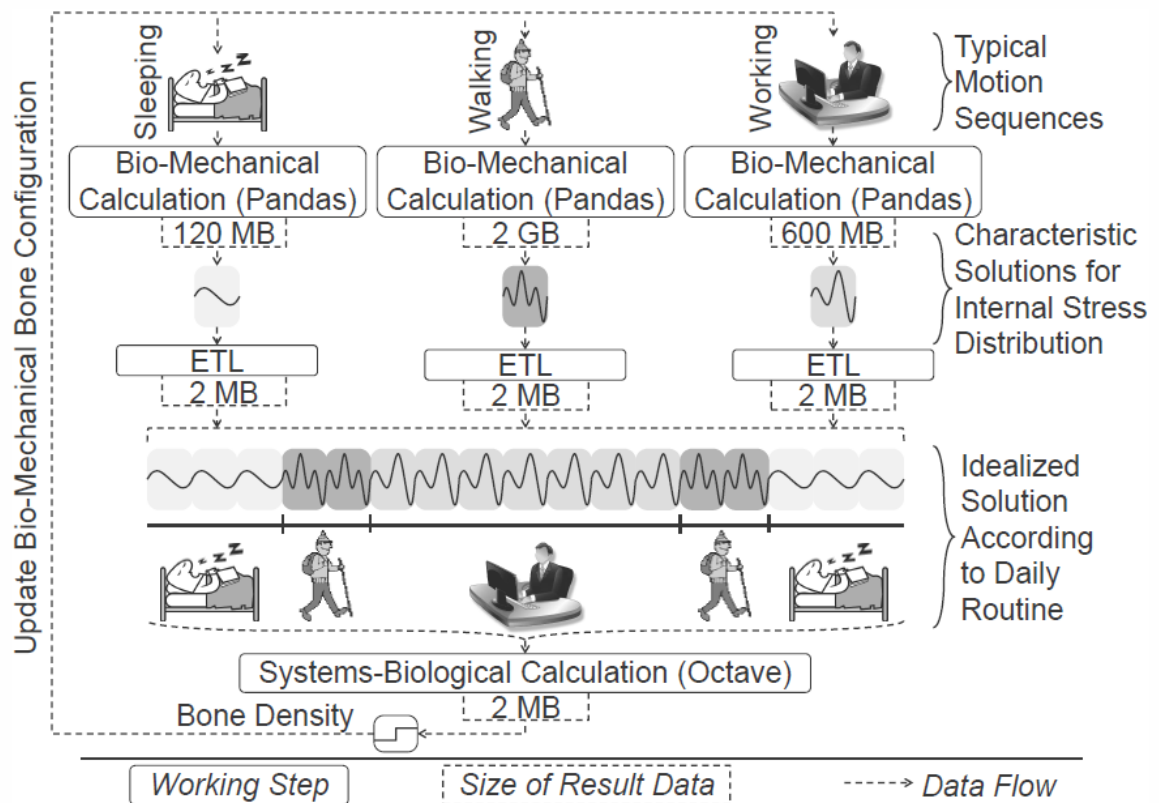
Abbildung 3.3: Gekoppelte Simulation von Strukturänderungen in Knochen Quelle: [RSM14b]
