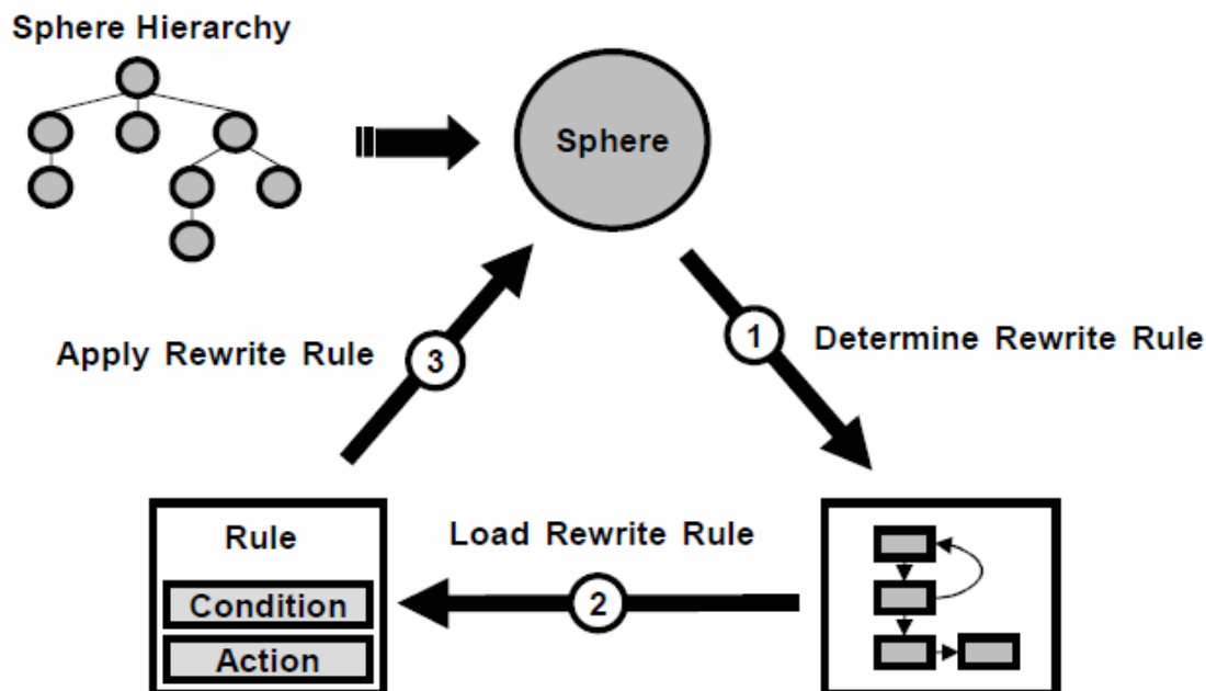
Abbildung 9.3: Ablauf der Optimierung Quelle: [VSS + 07]
