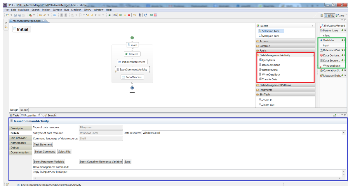
Abbildung 3.1: Data Management Aktivitäten im BPEL Designer
