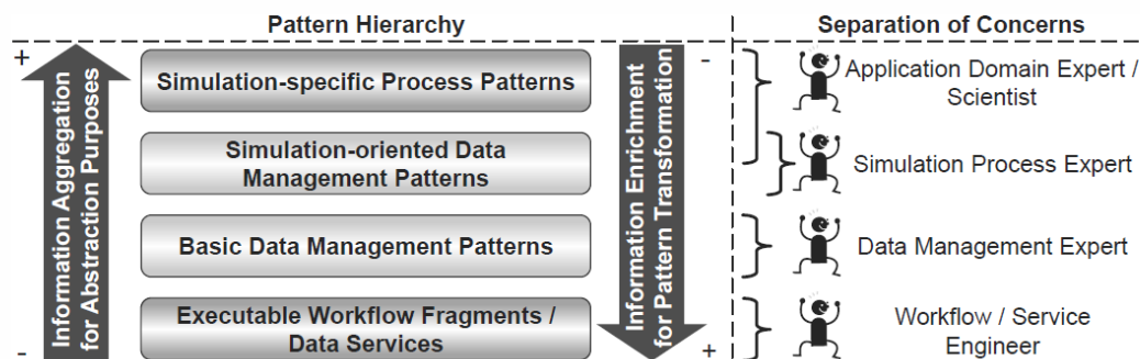
Abbildung 2.9: Hierarchie von Datenmanagementpatterns mit unterschiedlichen Abstraktionsebenen Quelle: [RSM14b]
