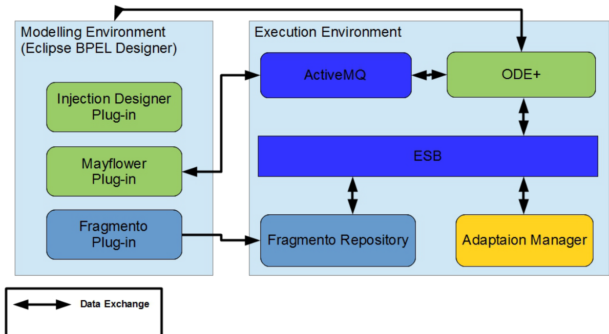
Abbildung 5.4: Architektur des Injektion Frameworks Quelle: [Bia14]
