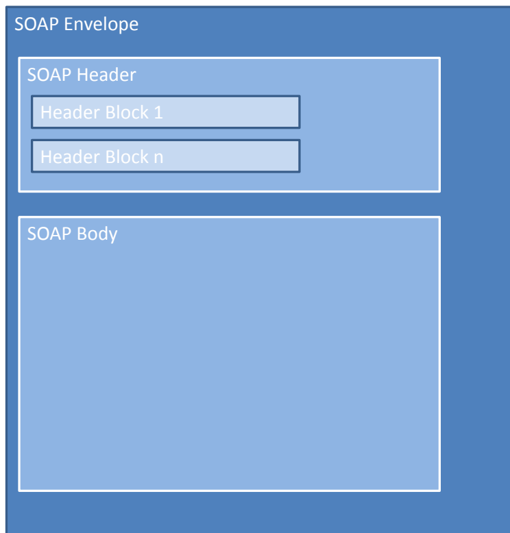
Abbildung 2.2: Aufbau einer SOAP Nachricht
