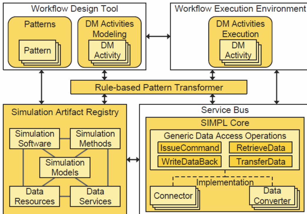
Abbildung 2.8: Das SIMPL-Rahmenwerk eingebettet in ein swfMS Quelle: [RRS + 11]
