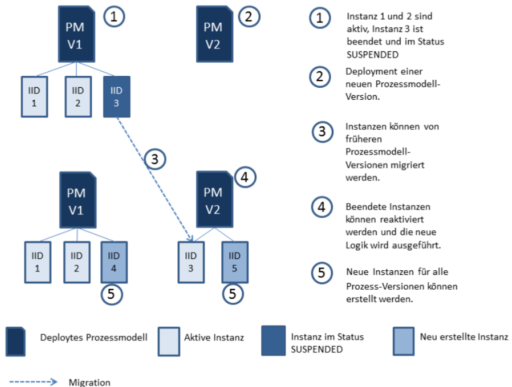
Abbildung 5.2: Hauptfunktionalitäten der Deploy New Version-Funktionalität Quelle: [Sch11]
