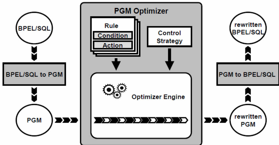
Abbildung 9.2: Ausführungsmodell Quelle: [VSS + 07]
