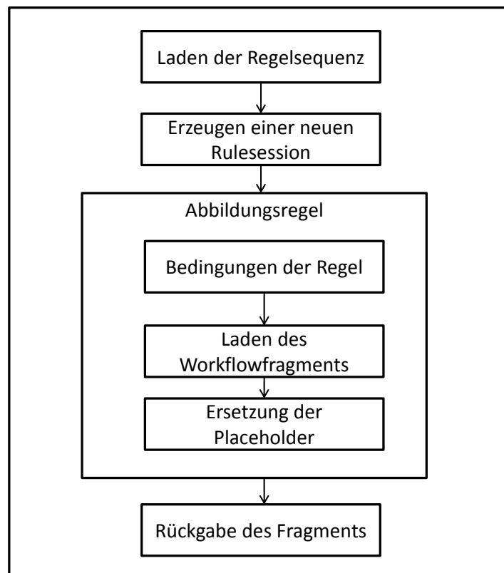
Abbildung 6.3: generischer Ablauf der Patterntransformation
