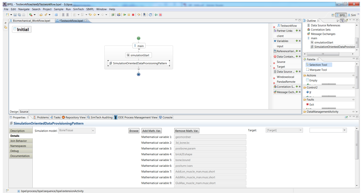
Abbildung 8.1: Testworkflow für die Messung des Anteils der Patterntransformation an der Datenbereitstellung
