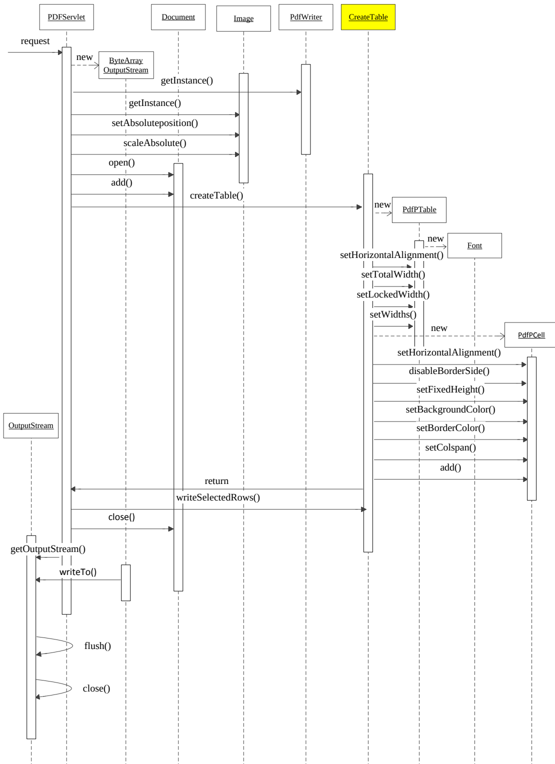
Abbildung 4.10: Sequenzdiagramm für die Generierung eines PDF-Dokumentes
