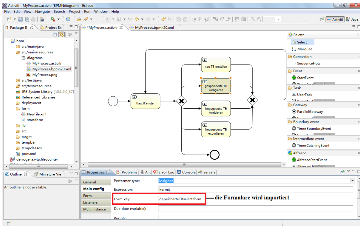
Abbildung 5.13: Implementierung des *.form-Files in der Aktivität durch Activiti Designer
