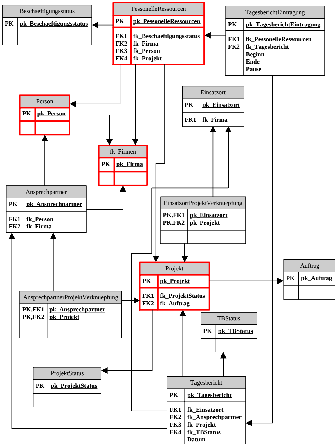
Abbildung 4.1: ER-Diagramm für die Datenbankstruktur
