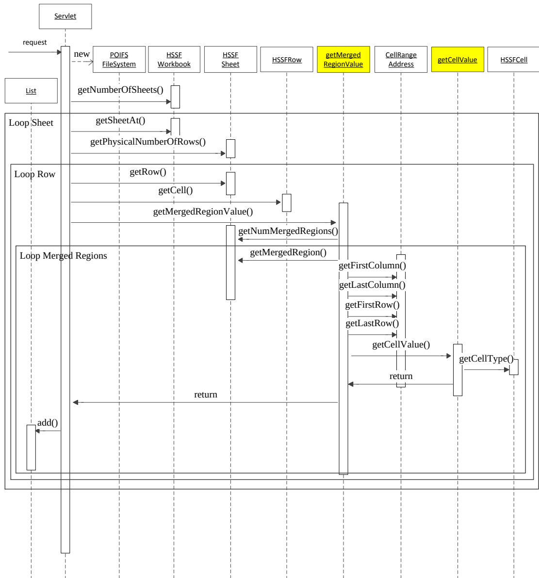
Abbildung 4.3: Sequenzdiagramm für das Lesen des Excel-Dokumentes durch Apache POI-HSSF
