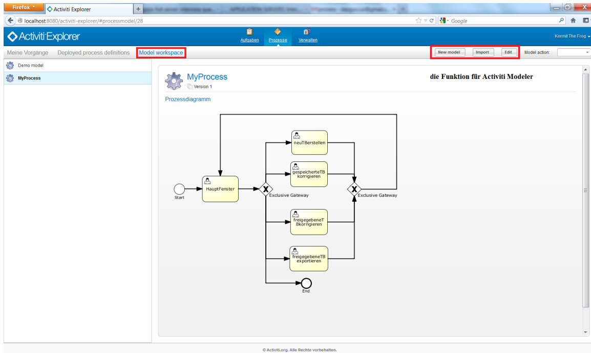
Abbildung 5.11: neue Funktion in Activiti Explorer
