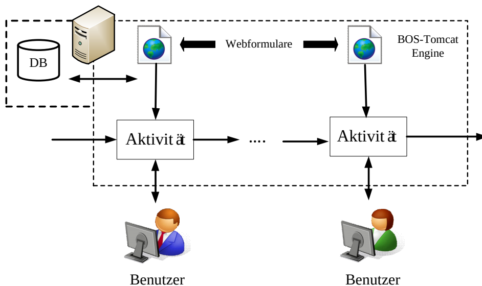
Abbildung 5.2: Beziehung zwischen BOS-Tomcat Engine und Benutzer
