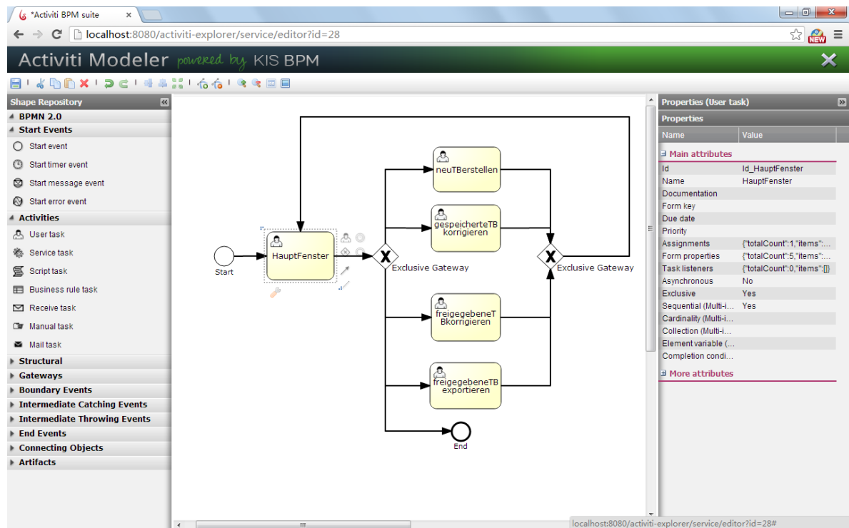
Abbildung 5.12: Erstellung des Prozessmodelles durch Activiti Modeler
