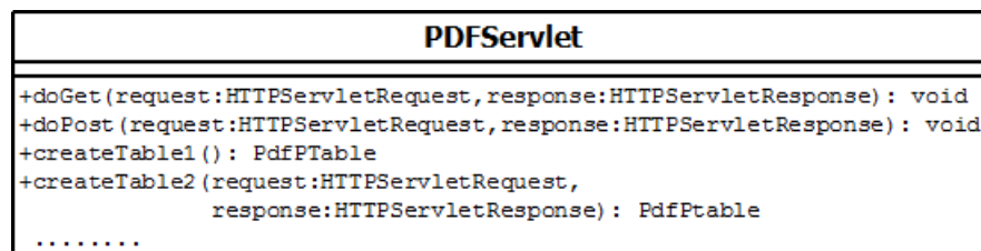
Abbildung 4.9: Klassendiagramm für die PDFServlet
