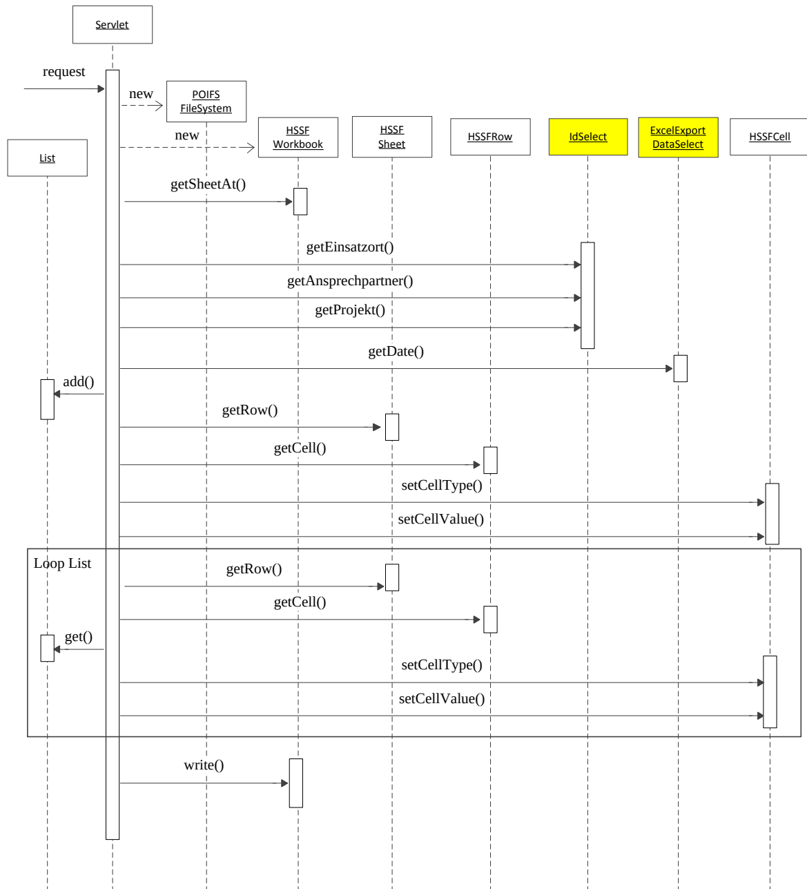
Abbildung 4.4: Sequenzdiagramm für das Schreiben in das Excel-Dokument durch Apache POI-HSSF
