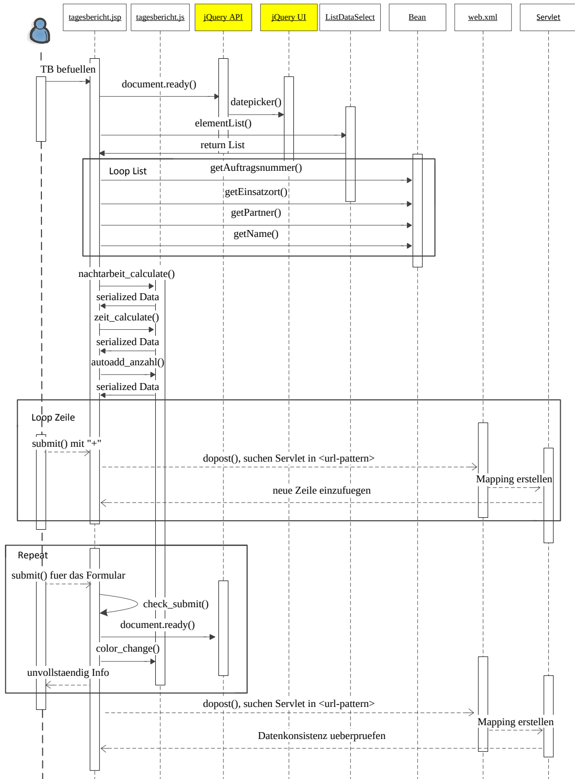
Abbildung 4.5: Sequenzdiagramm für die Funktionen der Benutzeroberflächen
