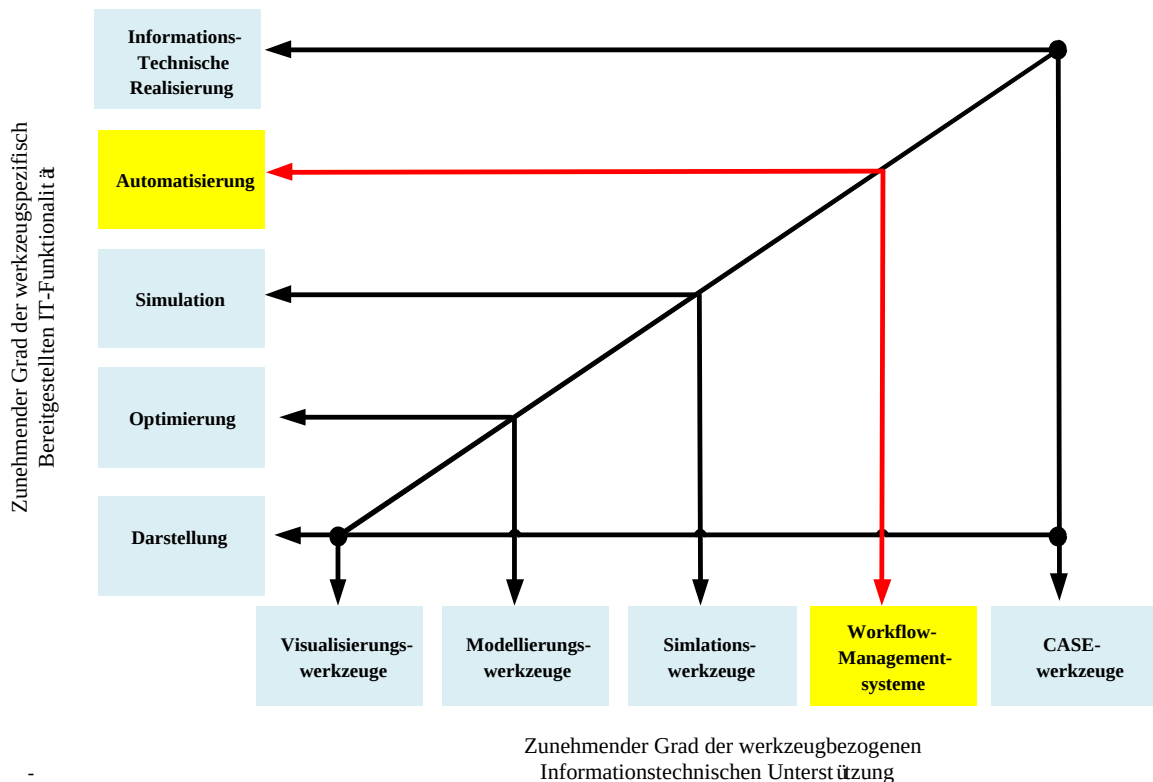
Abbildung 2.1: Prozessmanagement-Werkzeuge [NS02, S.201-210]
