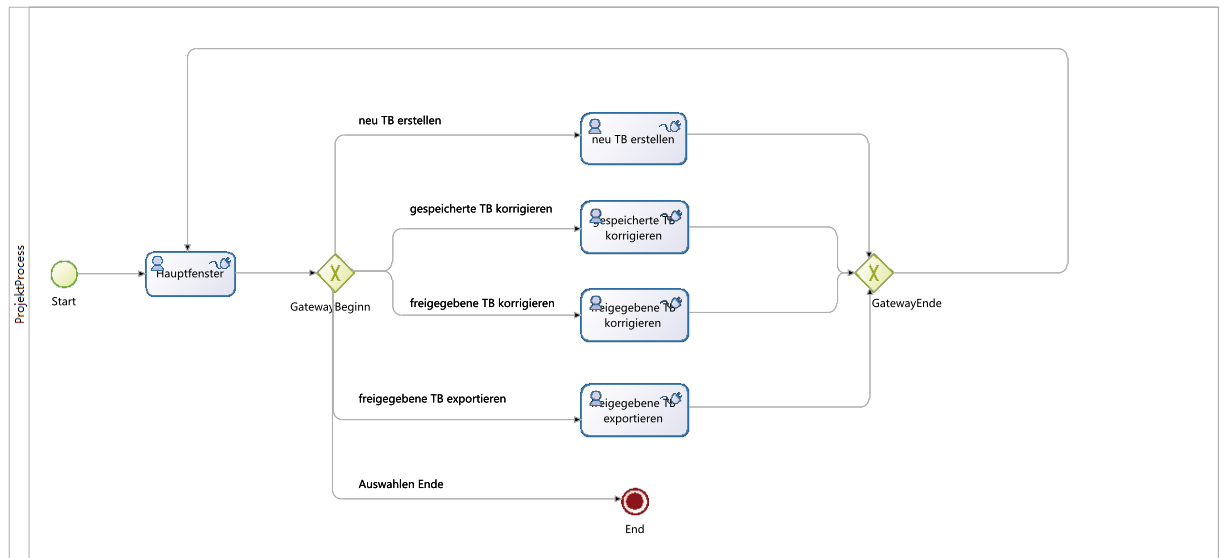
Abbildung 5.3: Beispielprozessmodell für die Bearbeitung des Tagesberichtes
