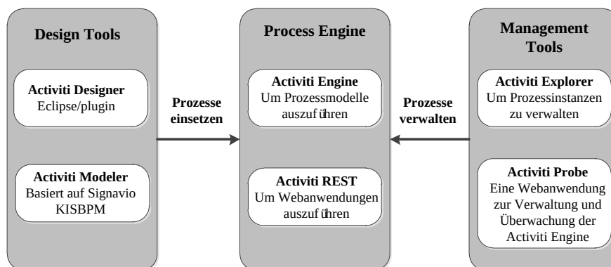
Abbildung 5.10: Komponenten der Activiti [Rad12, S.4]
