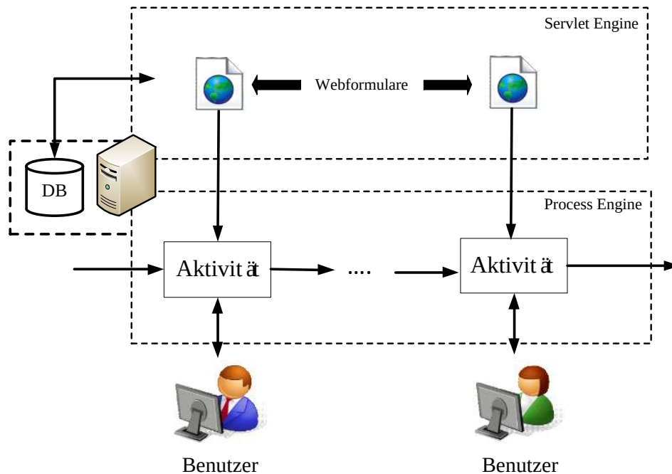
Abbildung 5.1: Beziehung zwischen den zwei Engines und den Benutzer
