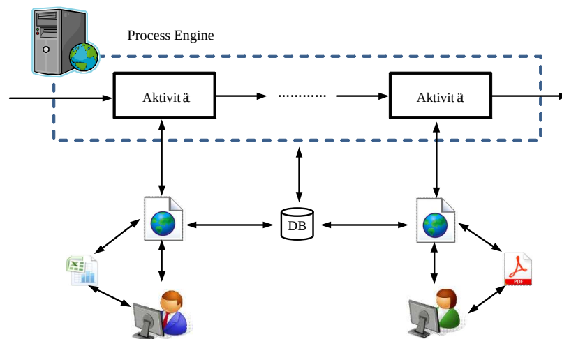
Abbildung 1.2: Beziehung zwischen den Benutzeroberflächen, der Process Engine und der Datenbank
