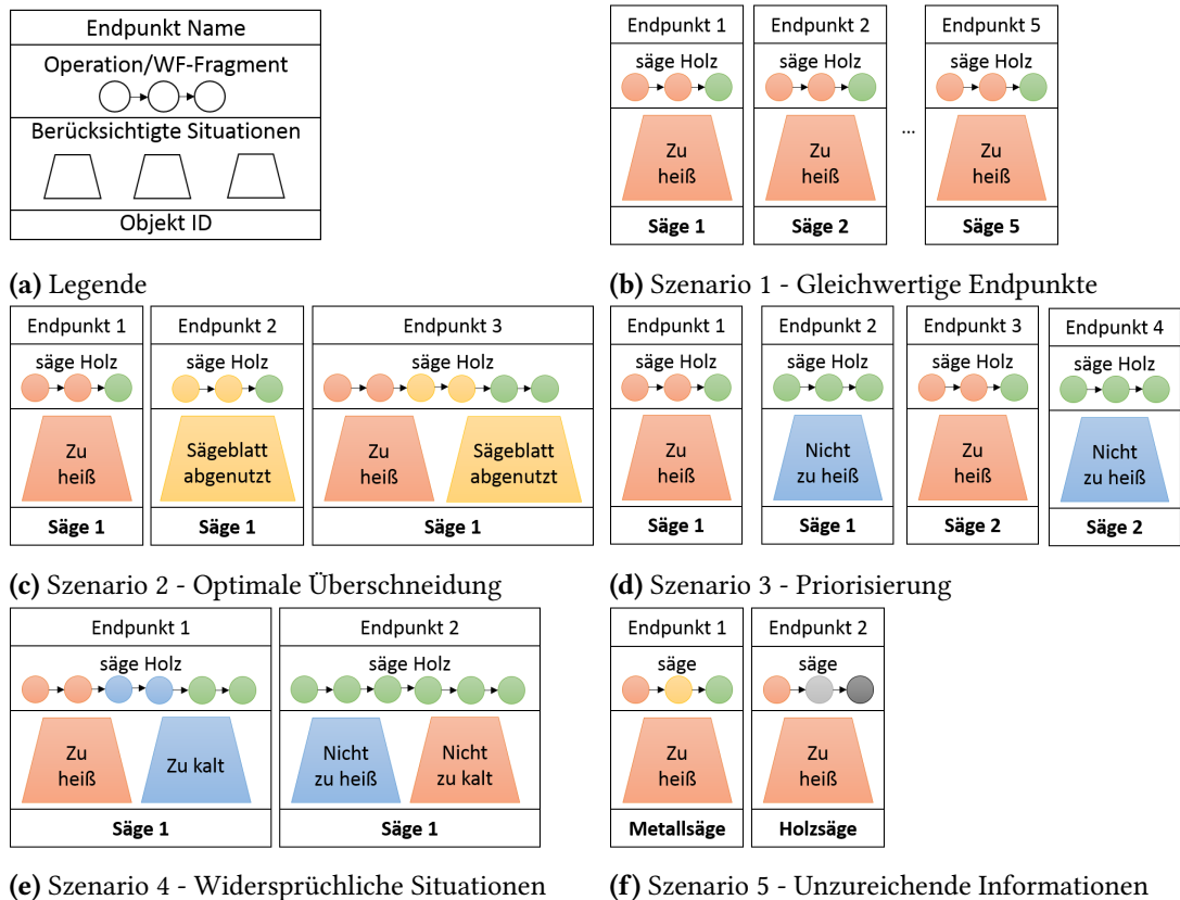
Abbildung 4.4.: Verschiedene Szenarien mit mehreren Endpunkten zur Auswahl
