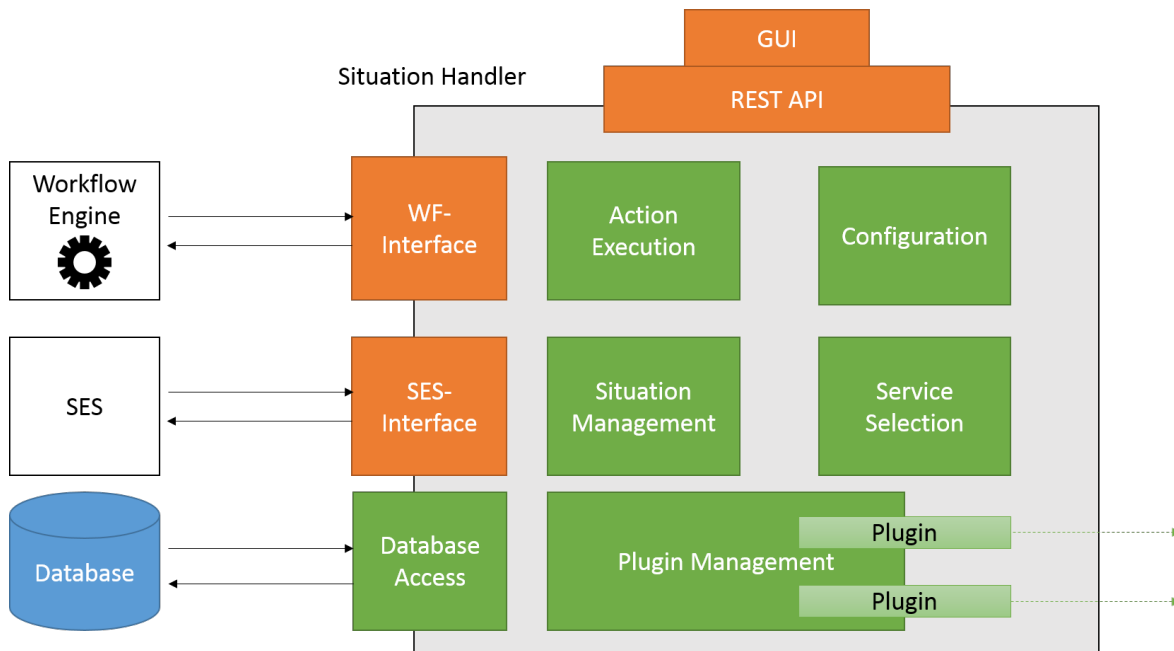
Abbildung 5.5.: Die Architektur des Situation Handlers.
