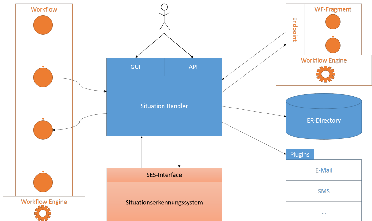
Abbildung 4.1.: Übersicht über die Integration des Situation Handlers.
