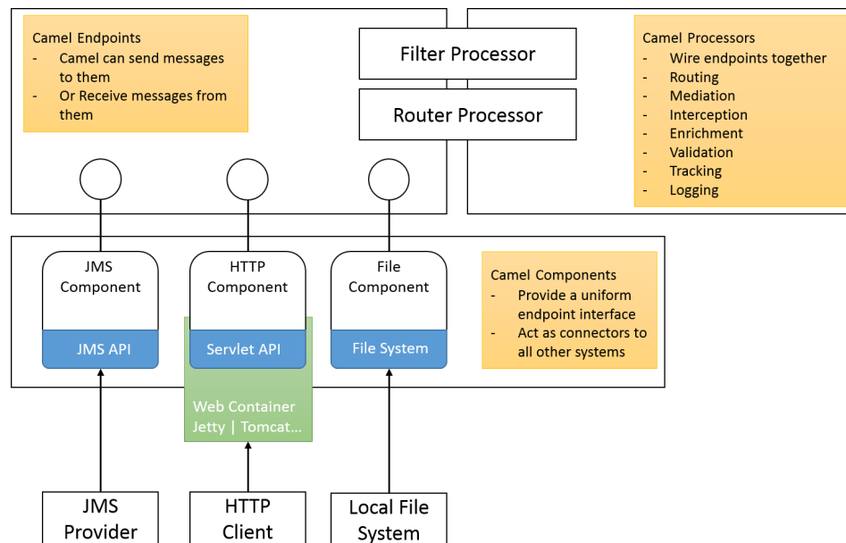
Abbildung 5.1.: Architektur Apache Camel [Apa]
