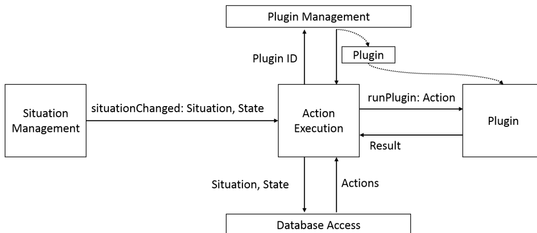
Abbildung 5.9.: Interaktion der Action-Execution-Komponente mit anderen Komponenten
