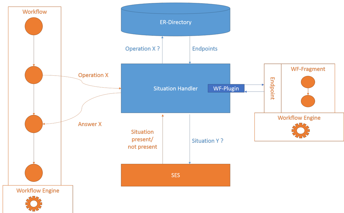
Abbildung 4.3.: Grafische Darstellung der Auswahl eines Operationsendpunktes.
