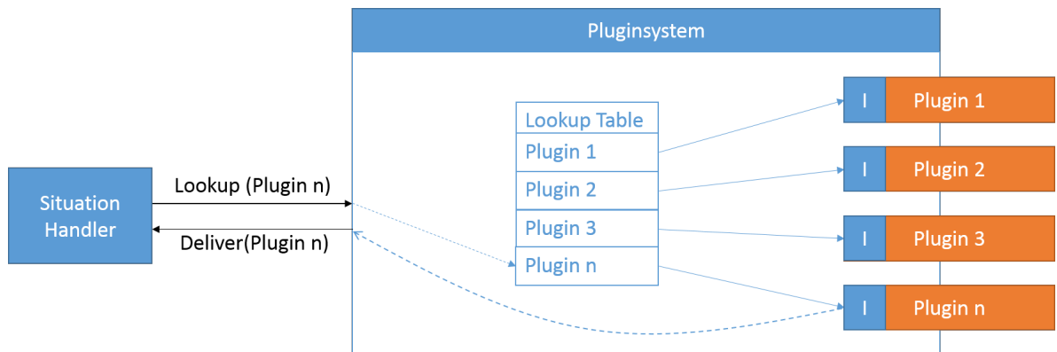
Abbildung 4.7.: Pluginsystem und dessen Verwendung.
