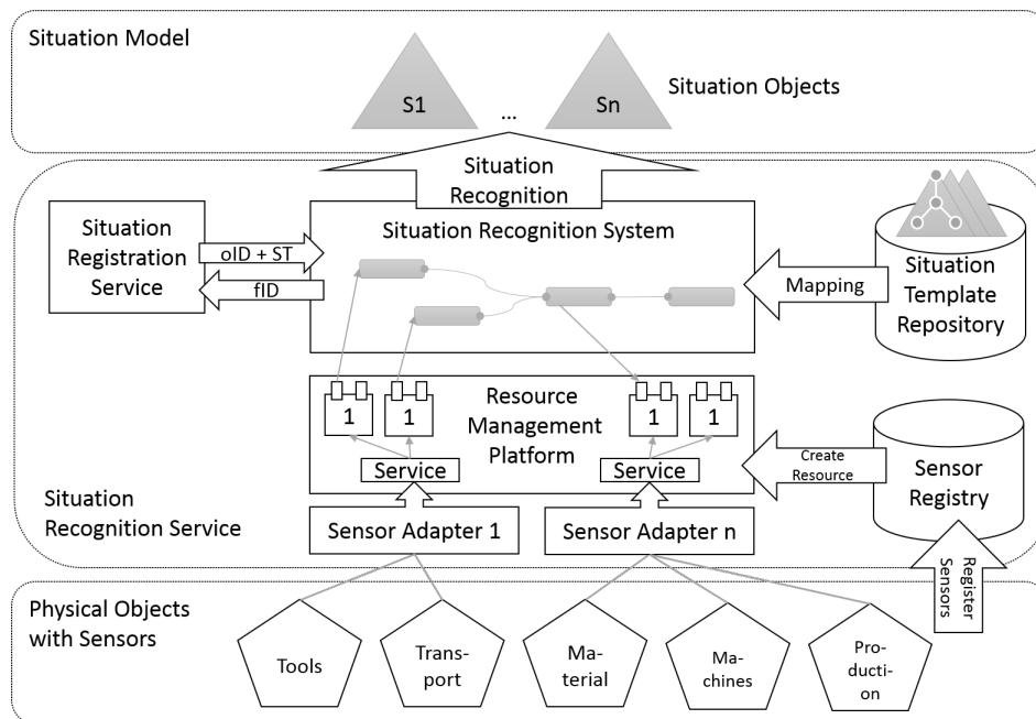
Abbildung 3.4.: SitRS - Architektur [HWS + 15]
