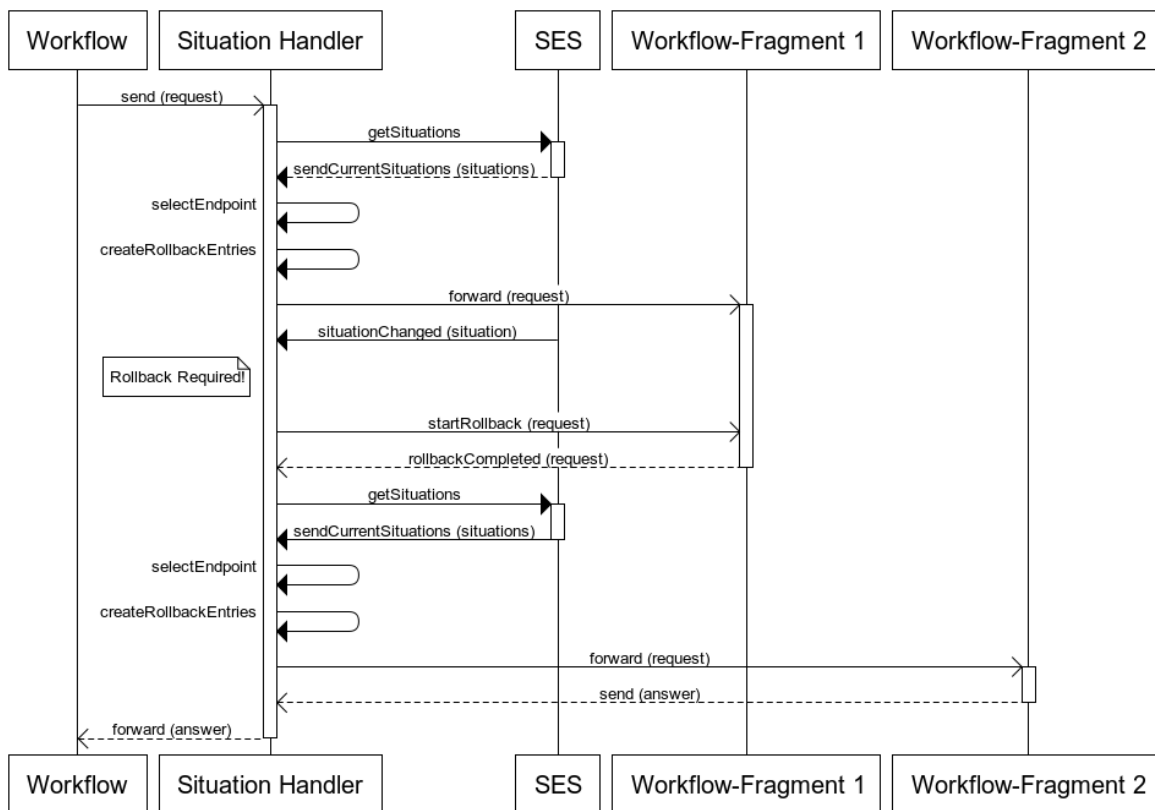
Abbildung 4.6.: Die Prozedur bei einem situationsbedingten Rollback, einschließlich den Kommunikationsbeziehungen.
