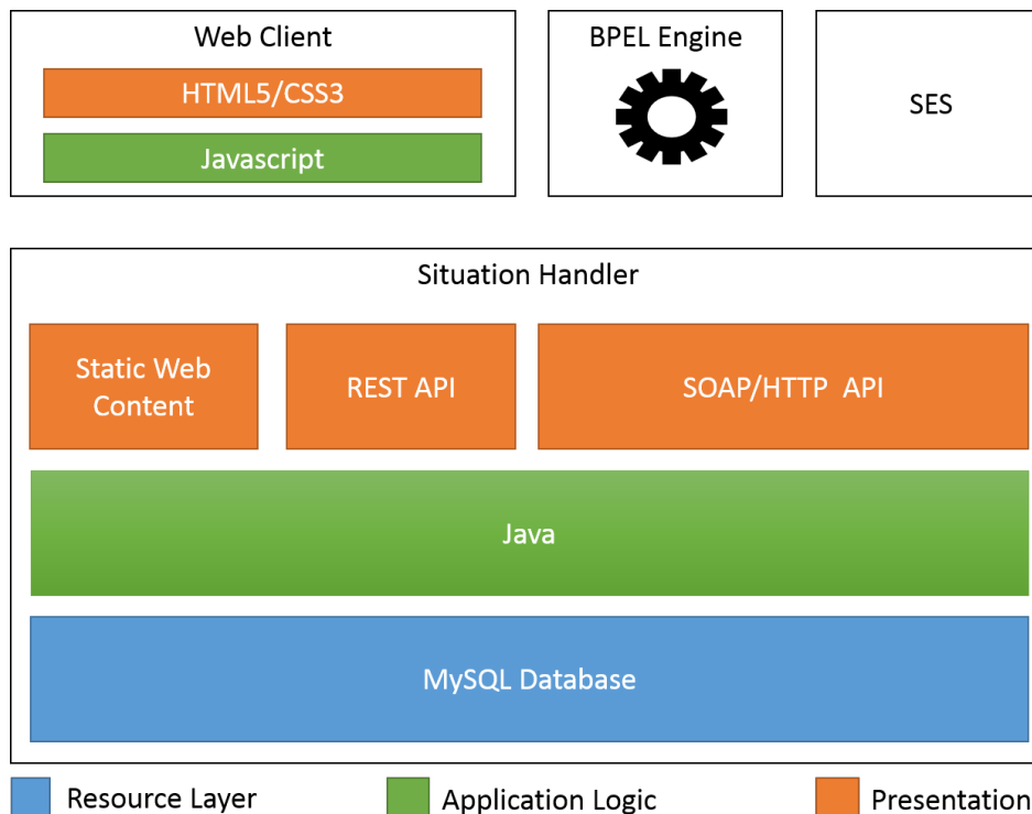
Abbildung 5.3.: Eingesetzte Technologien in der Drei-Schichten-Architektur des Situation Handlers
