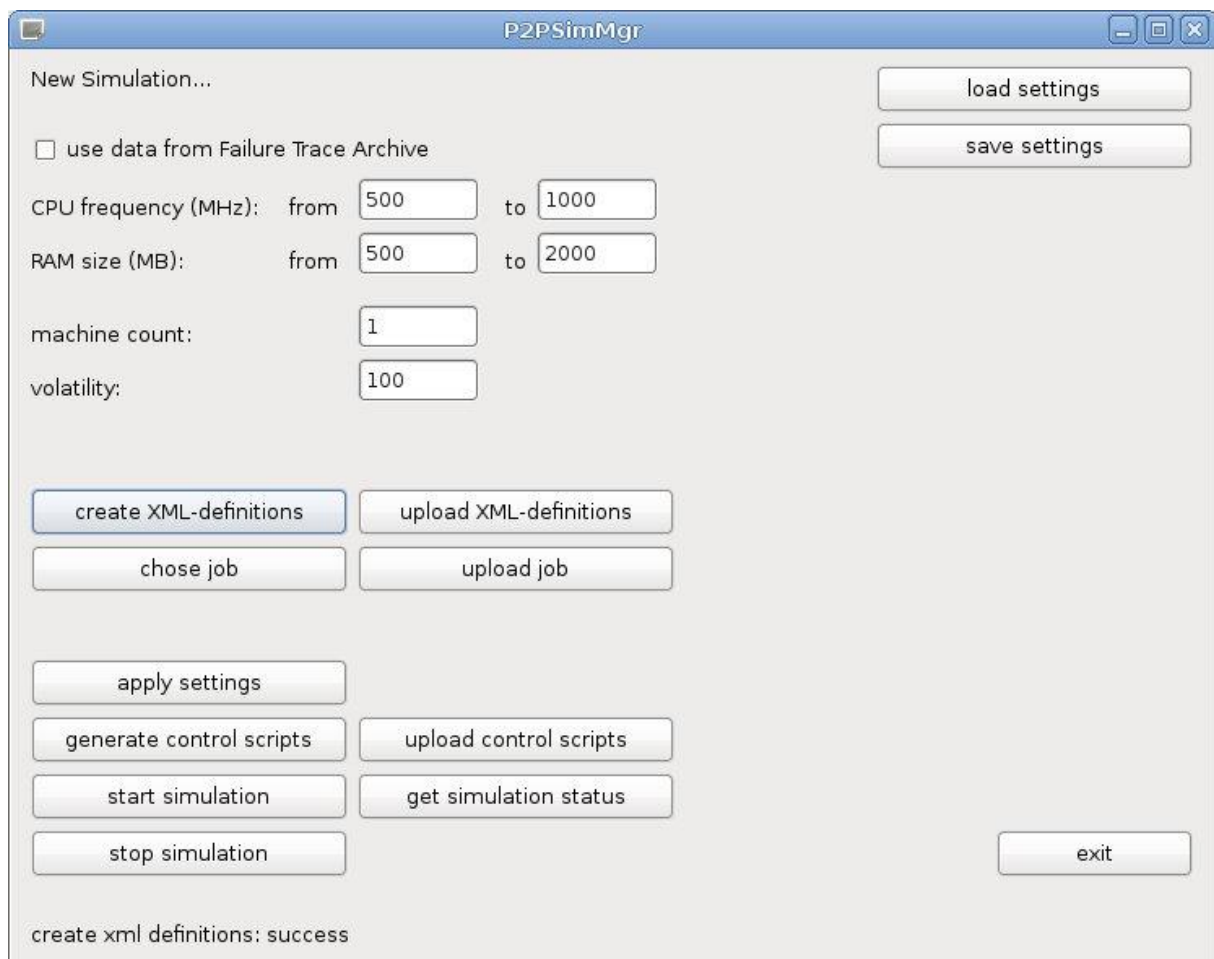
Abbildung 7: Grafische Benutzerschnittstelle
