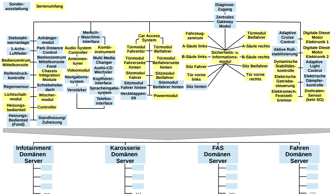
Abbildung 1.2.: Domänenserver-Architektur im Fahrzeug nach [MKS12]
