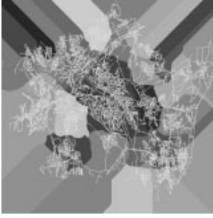
Abb. 8.11: Regioneneinteilung (Pseudograustufen)
