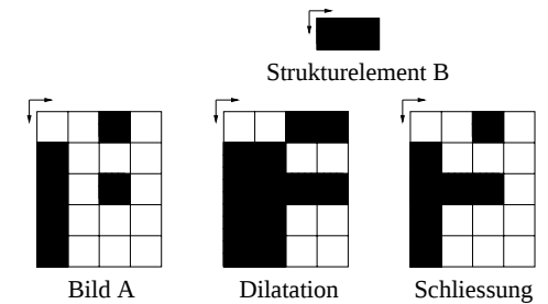
Abb. 8.4: Schließung
