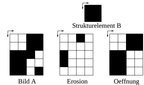
Abb. 8.5: Öffnung
