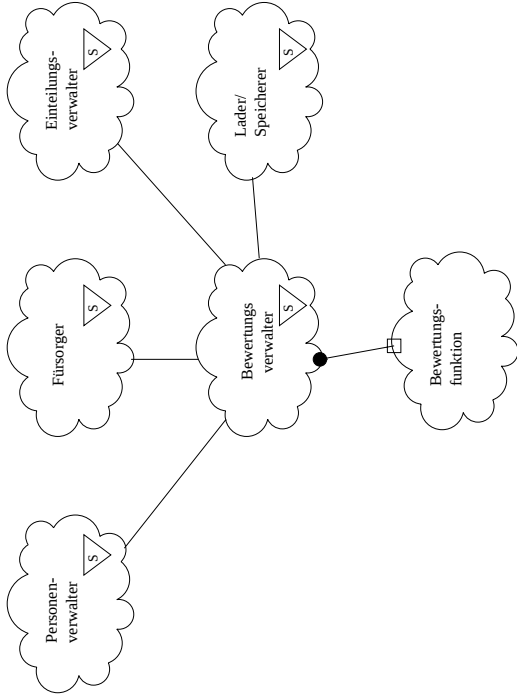
Abb. 5.9: Bewertungsverwalter
